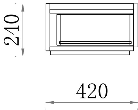
側視圖
