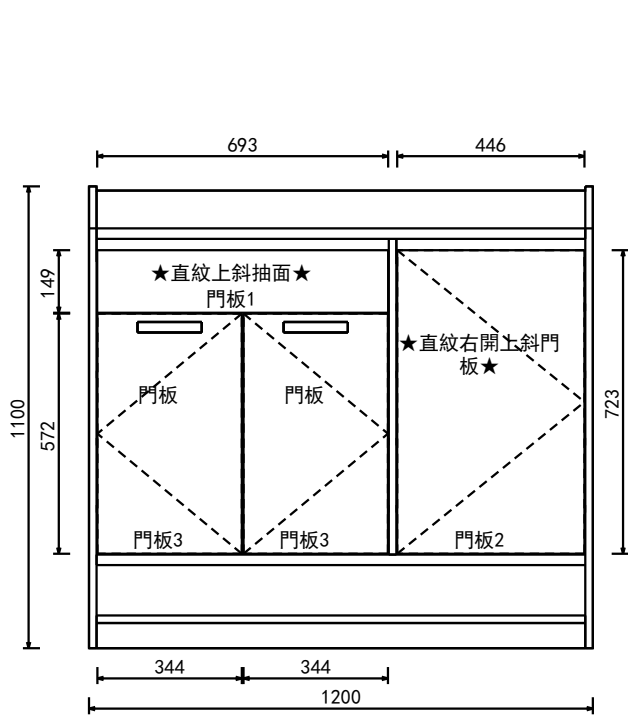
立面圖
