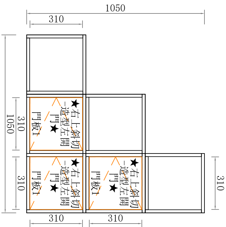
立面圖
