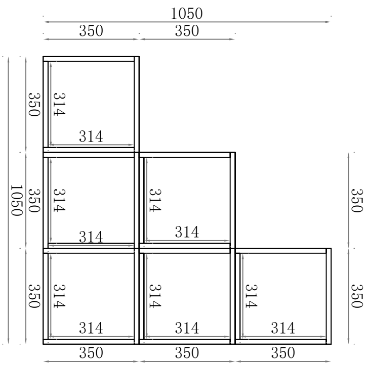
結構圖
