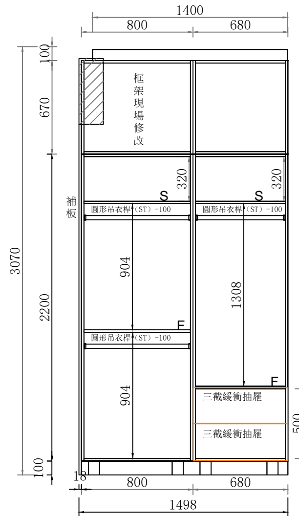
B向 結構圖
