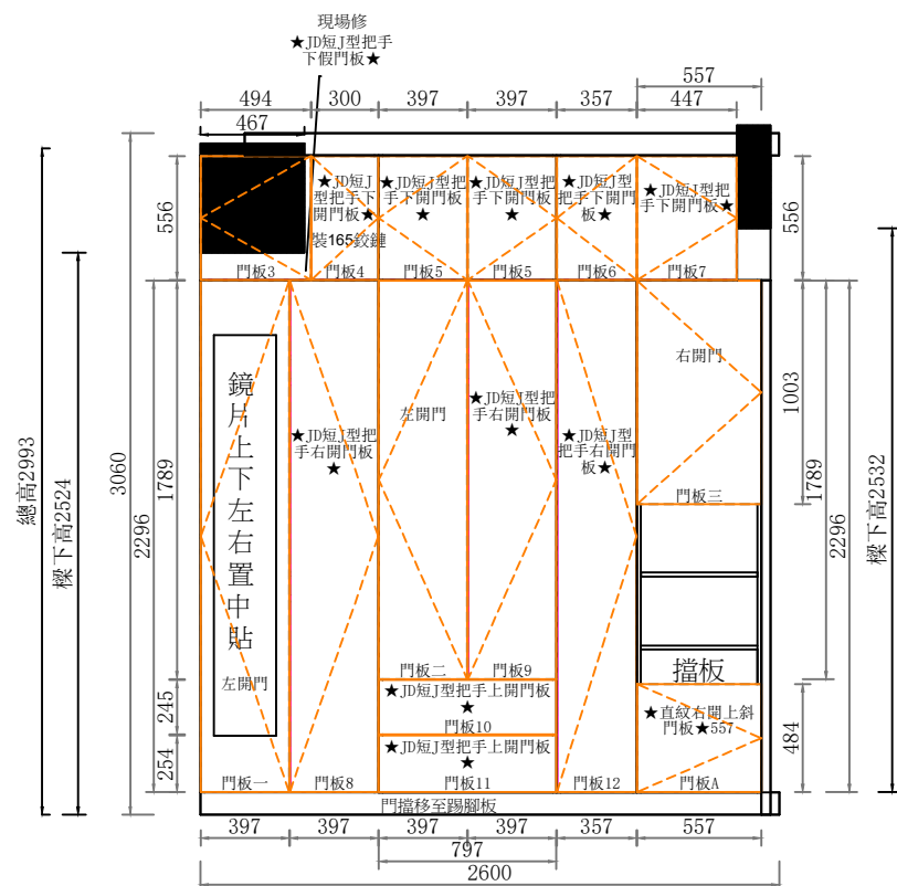
B向 立面圖
