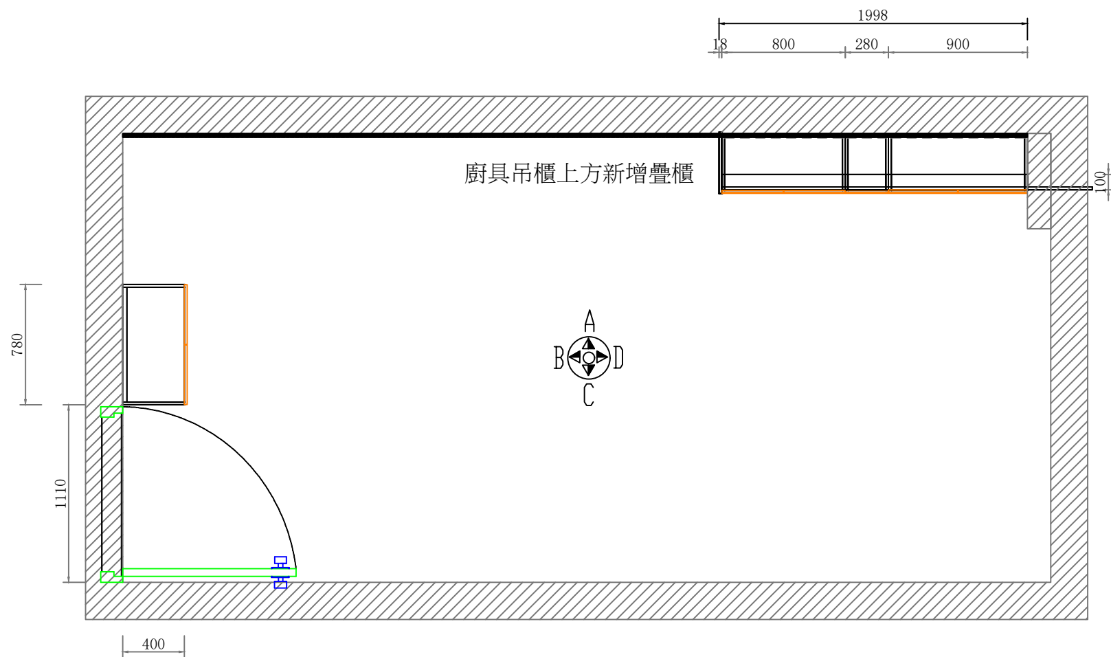
主臥頂櫃平面圖
