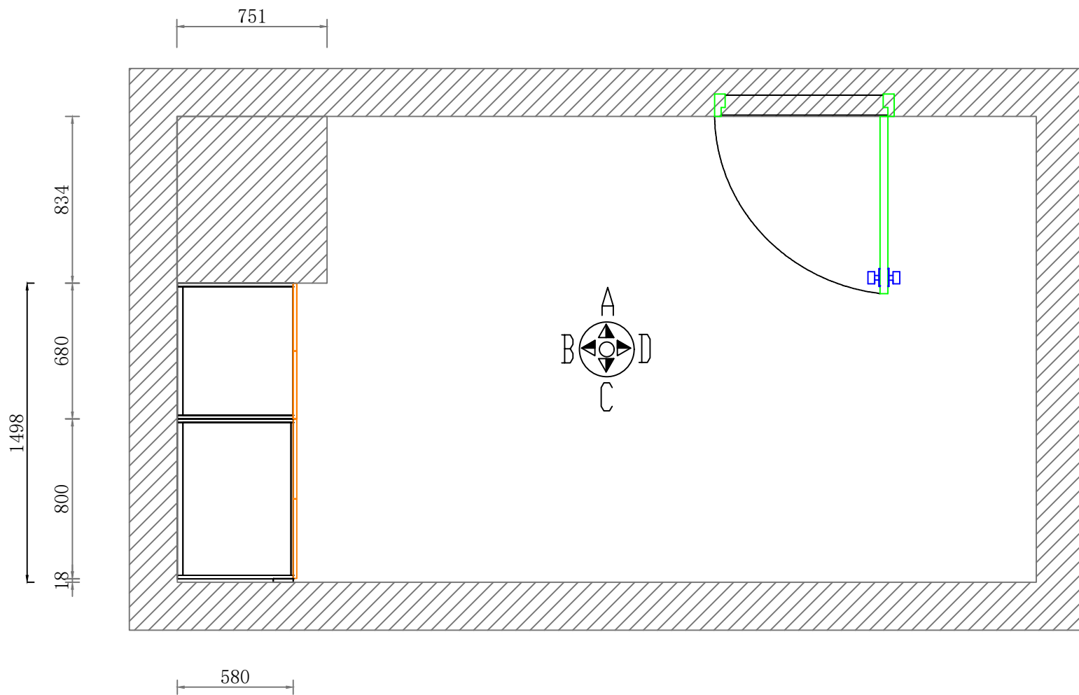
臥地櫃平面圖
