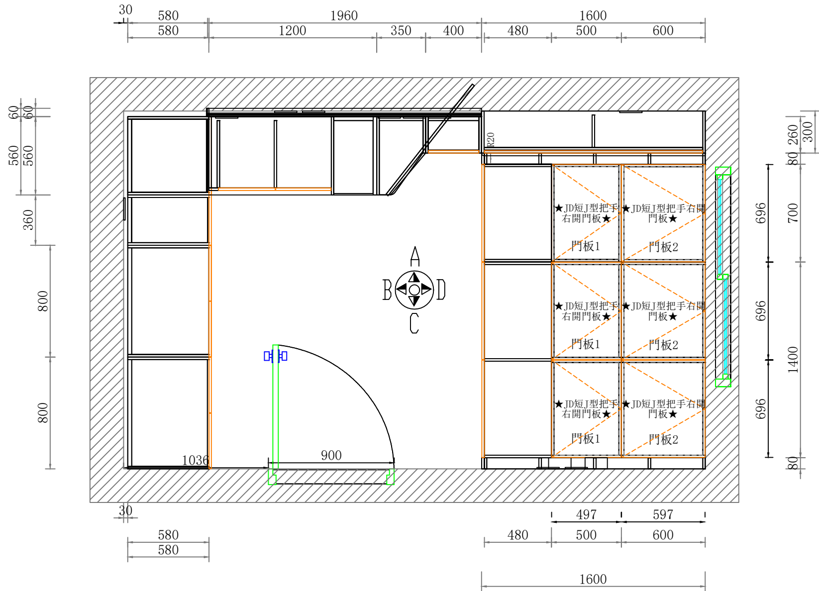
主臥地櫃平面圖
