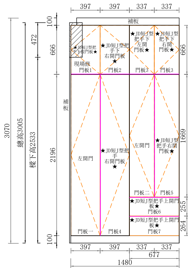
B向 立面圖
