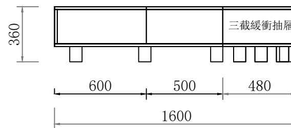
C向 結構圖
