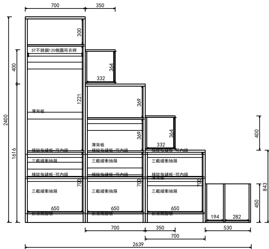
A向 結構圖
