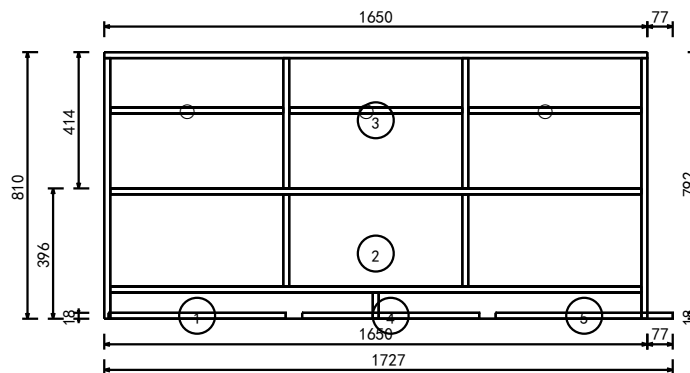
A向 結構圖
