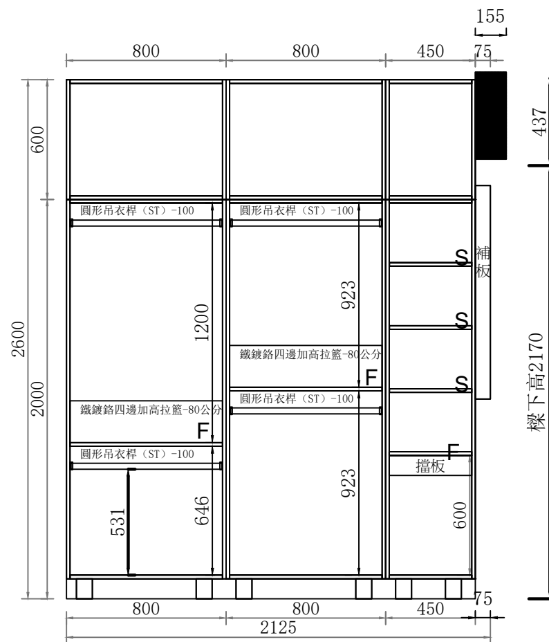
C向 結構圖
