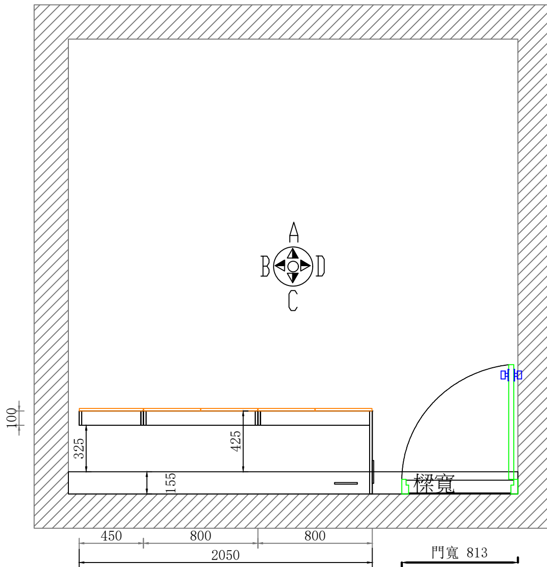
尚勇路23號頂櫃平面圖
