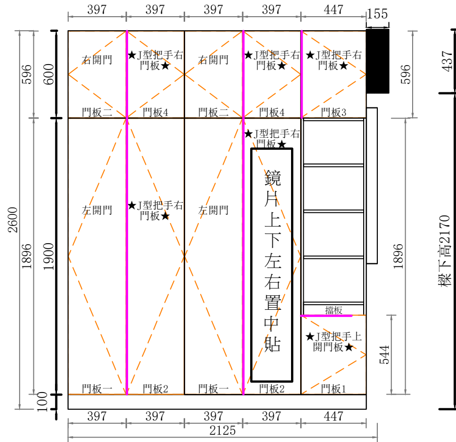
C向 立面圖
