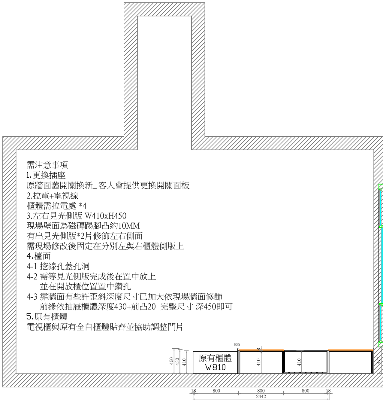
尚勇路客廳_追加電視櫃地櫃平面圖-1
