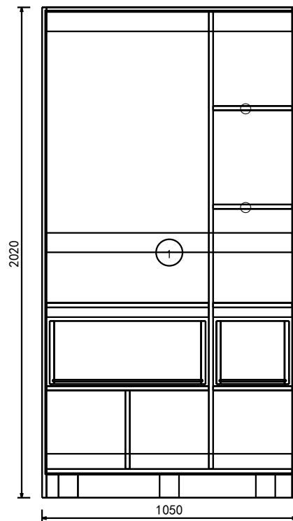
A向 結構圖
