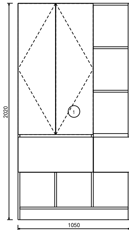
A向 外觀圖
