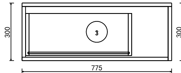
C向 結構圖
