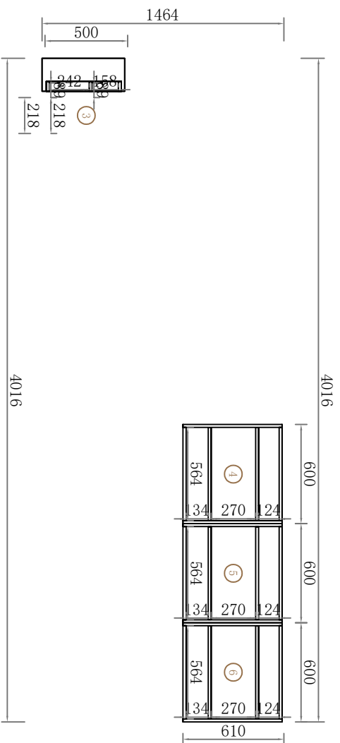
D向结构图
