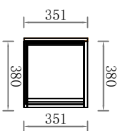
D向地柜平面图
