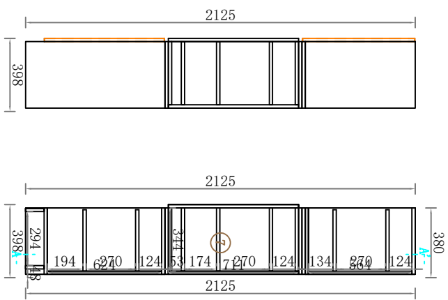
D向外观图 D向结构图
