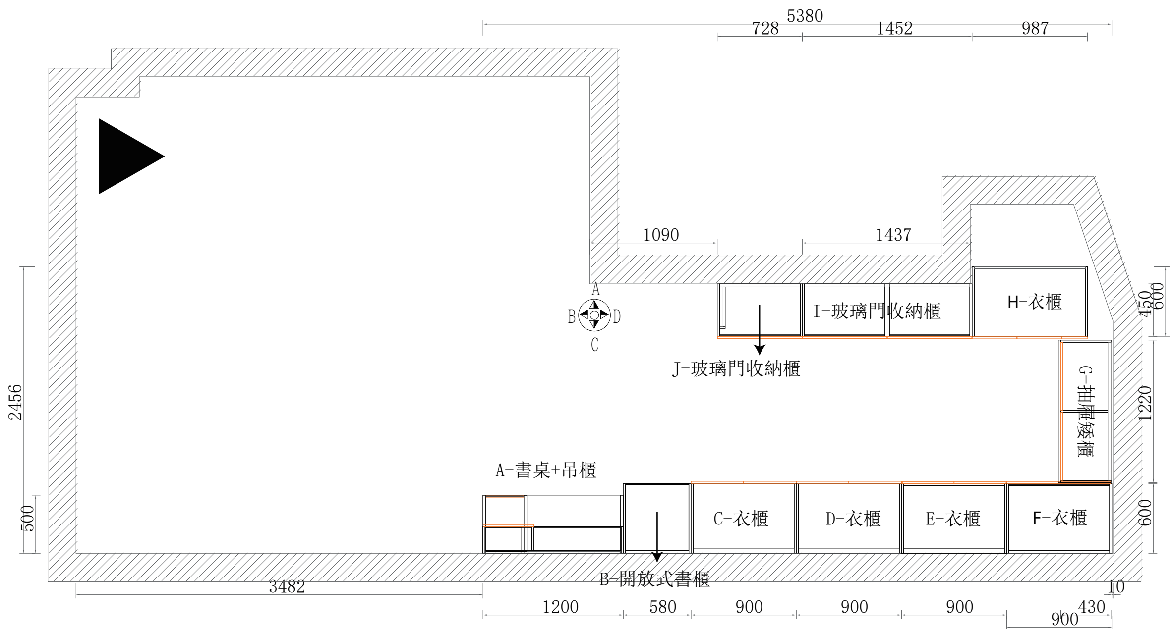
地櫃平面圖
