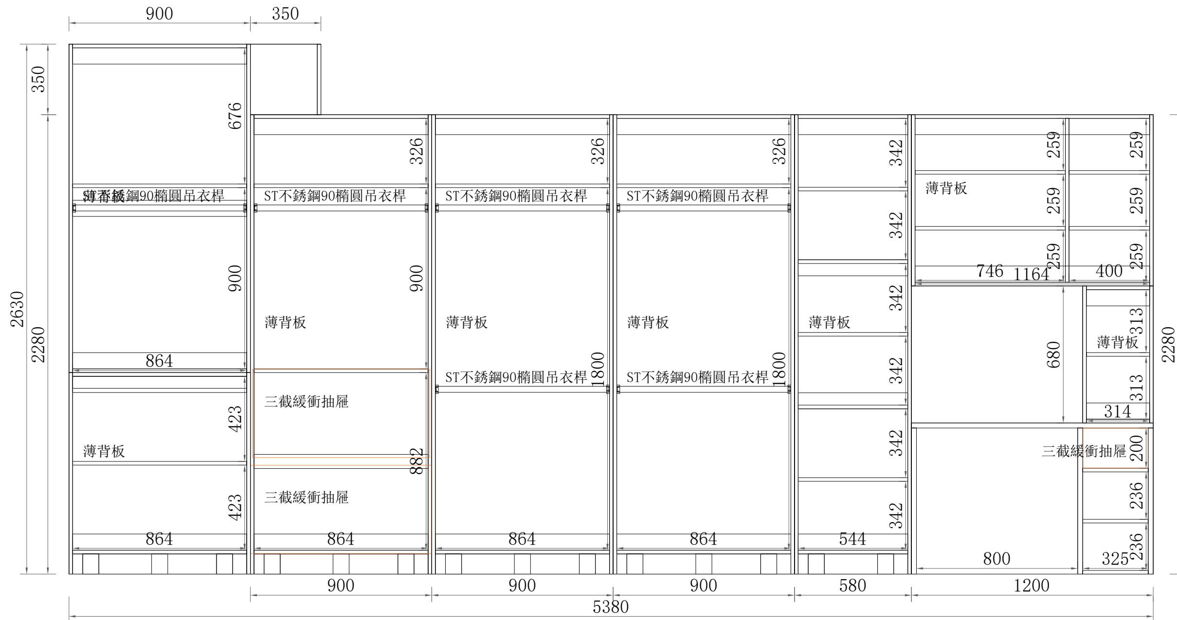
C向 結構圖
