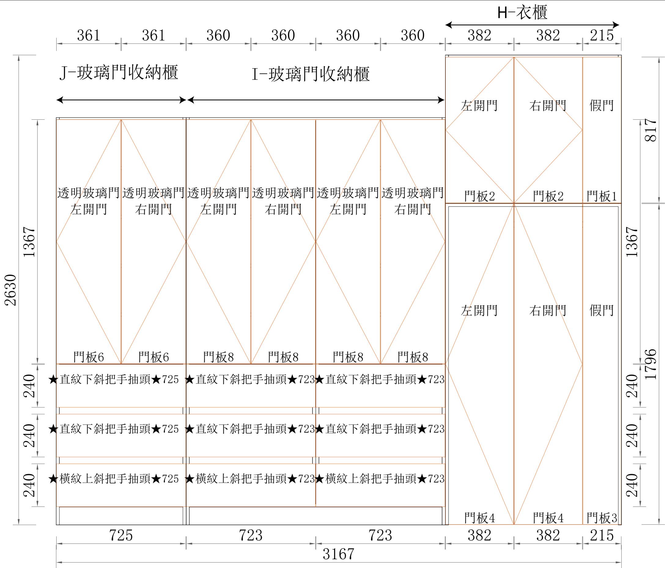
A向 立面圖
