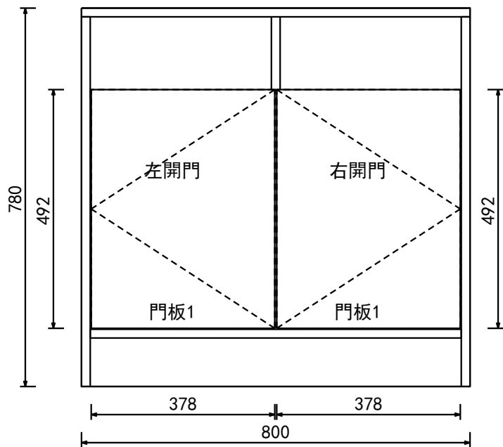
立面圖
