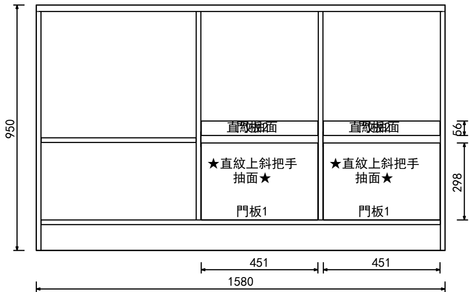
立面圖
