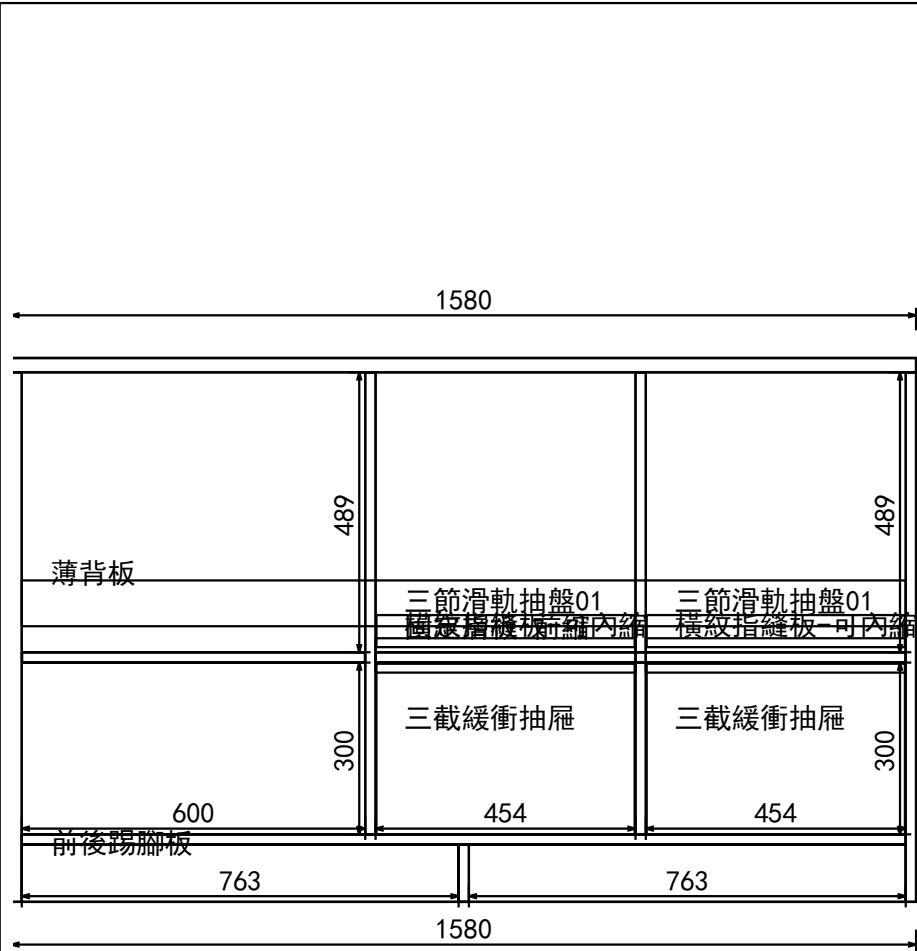
結構圖
