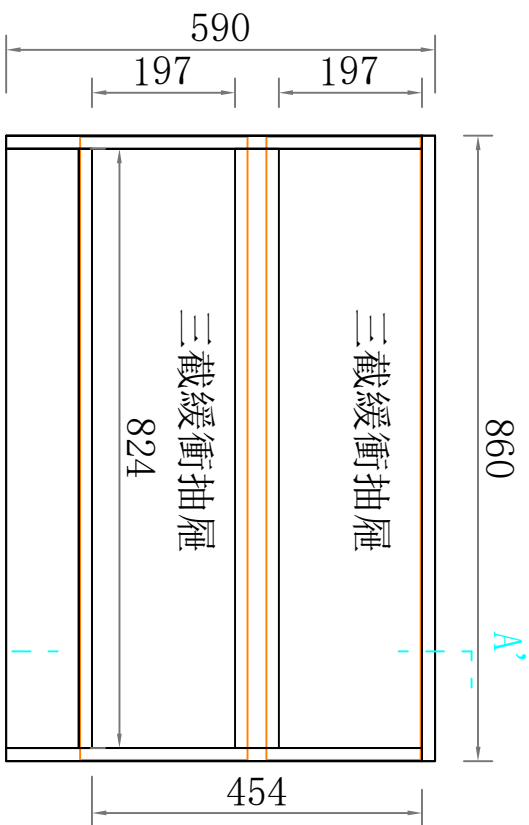
結構圖
