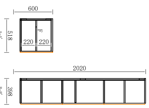
側視圖
