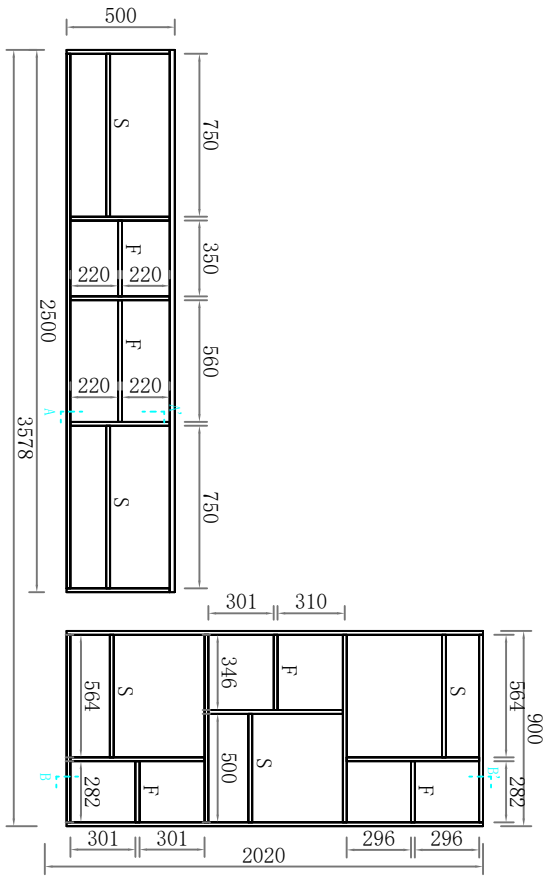
外觀圖
