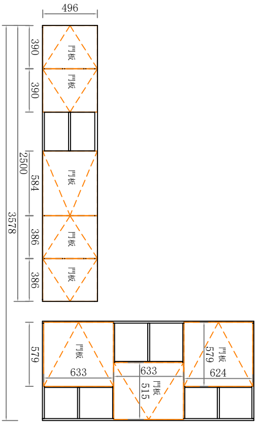
外觀圖
