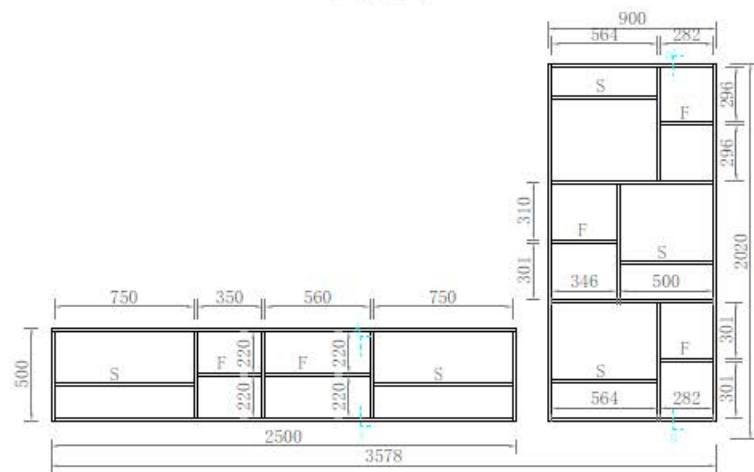
結構圖
