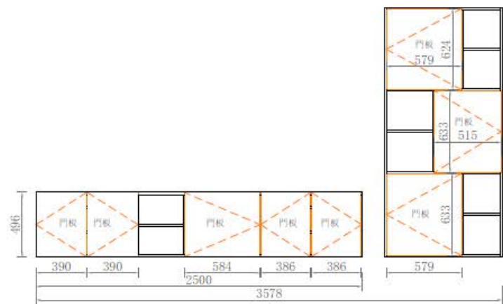
外觀圖
