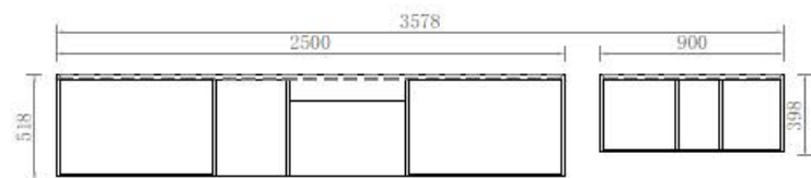
平面圖
