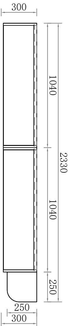
A向平面圖
