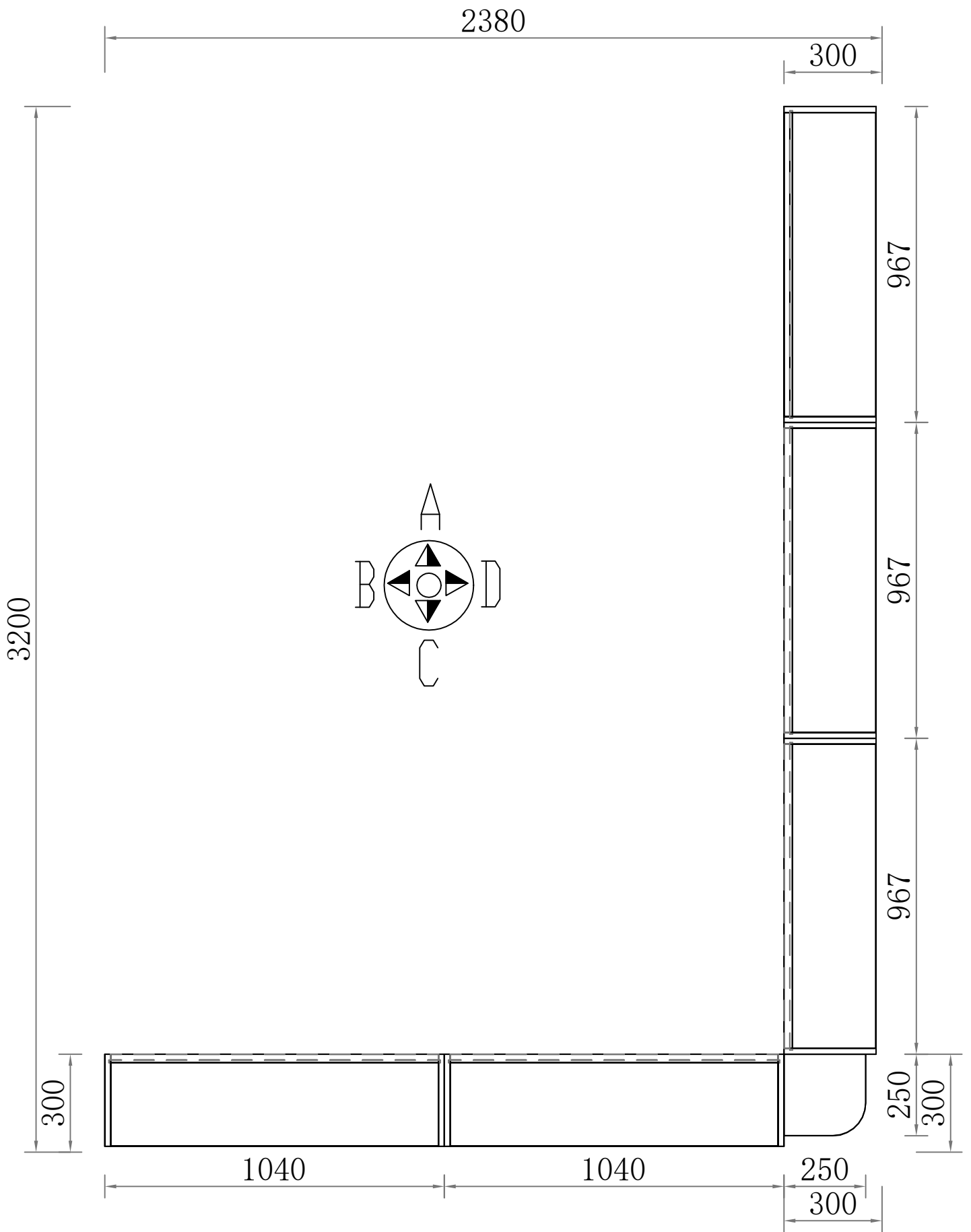
平面圖
