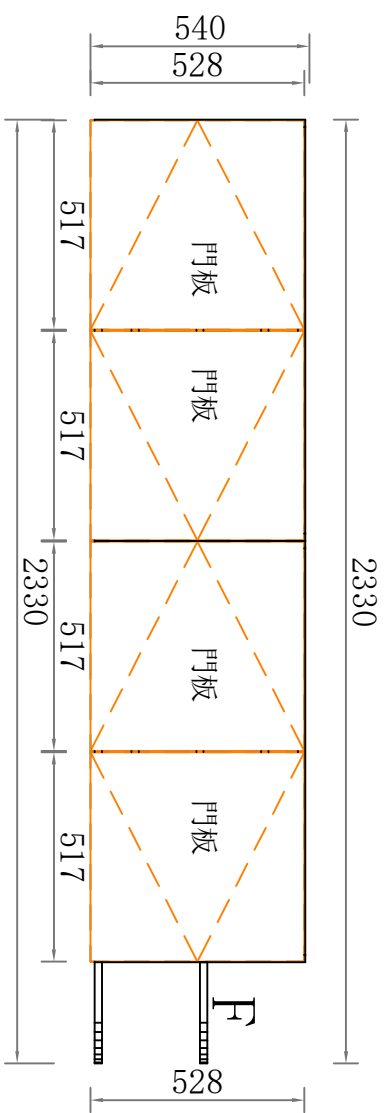
A向外觀圖
