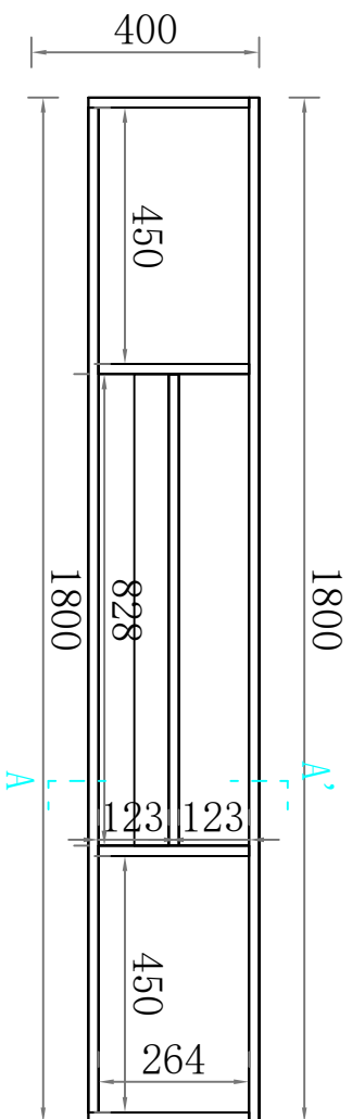
結構圖
