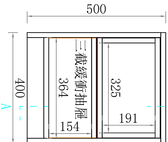
結構圖
