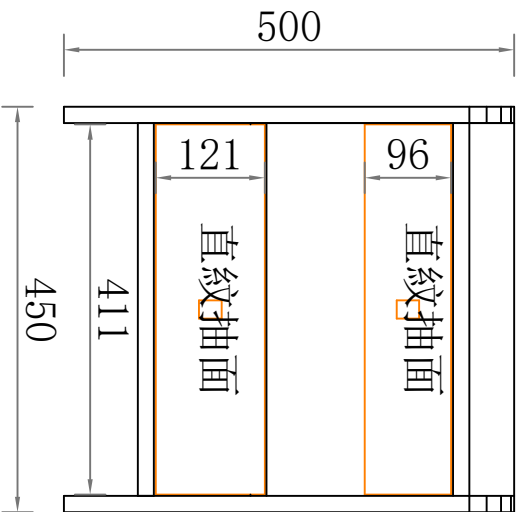
外觀圖
