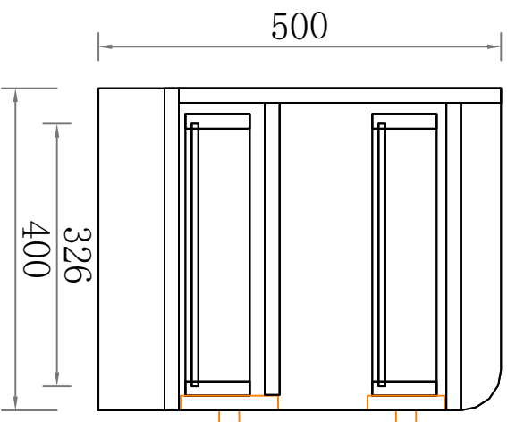
結構圖
