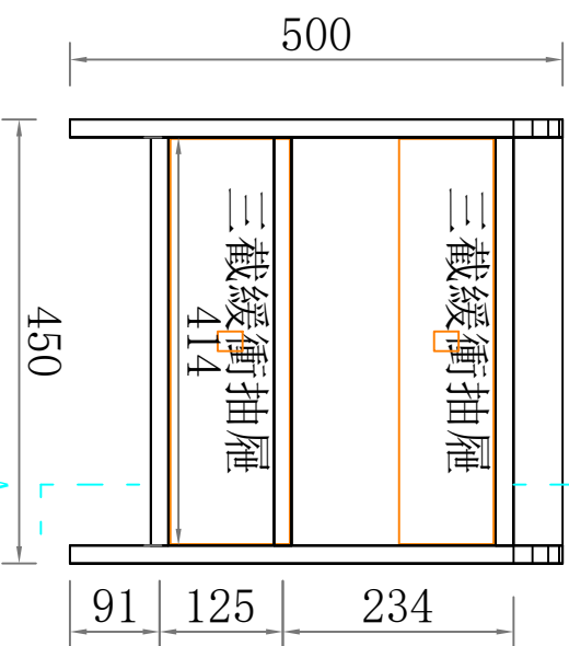
結構圖
