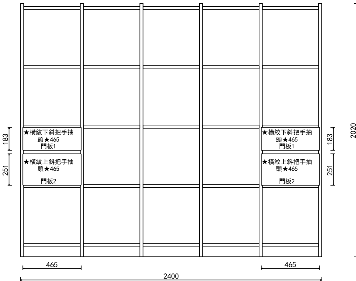
立面圖
