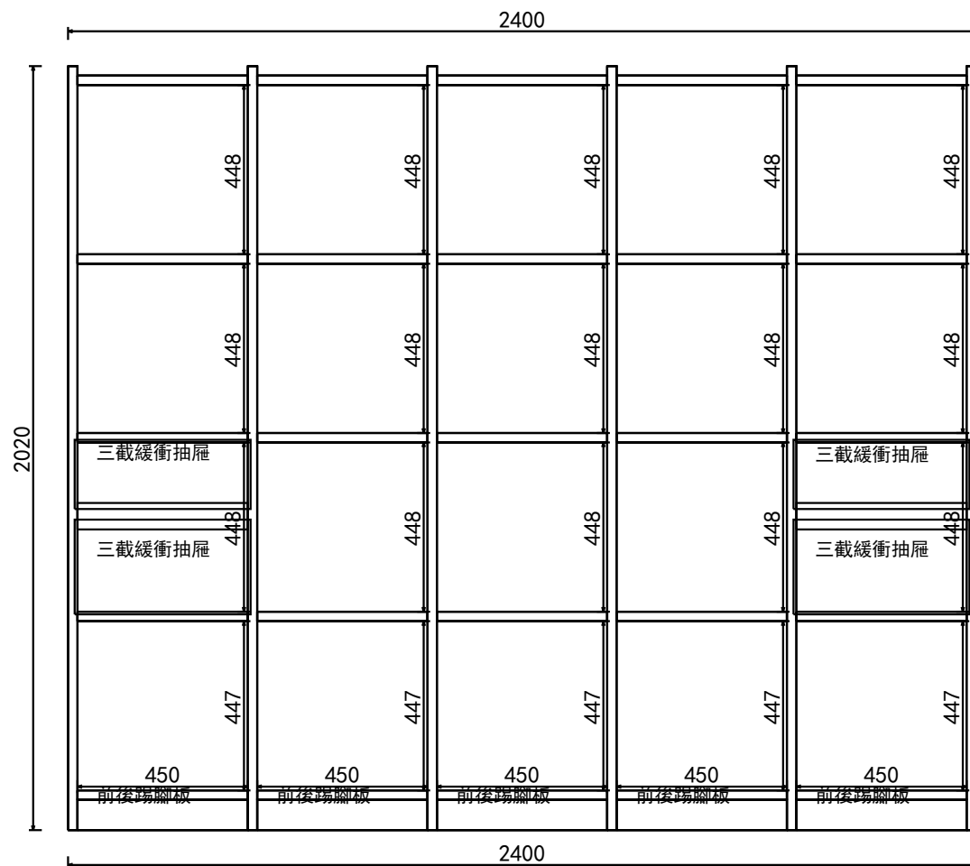
結構圖
