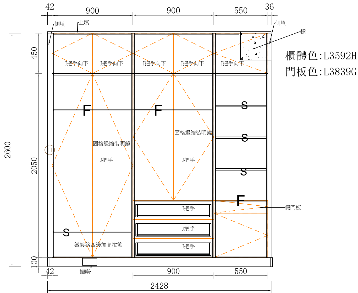
佳順大順女兒房A向立面圖
