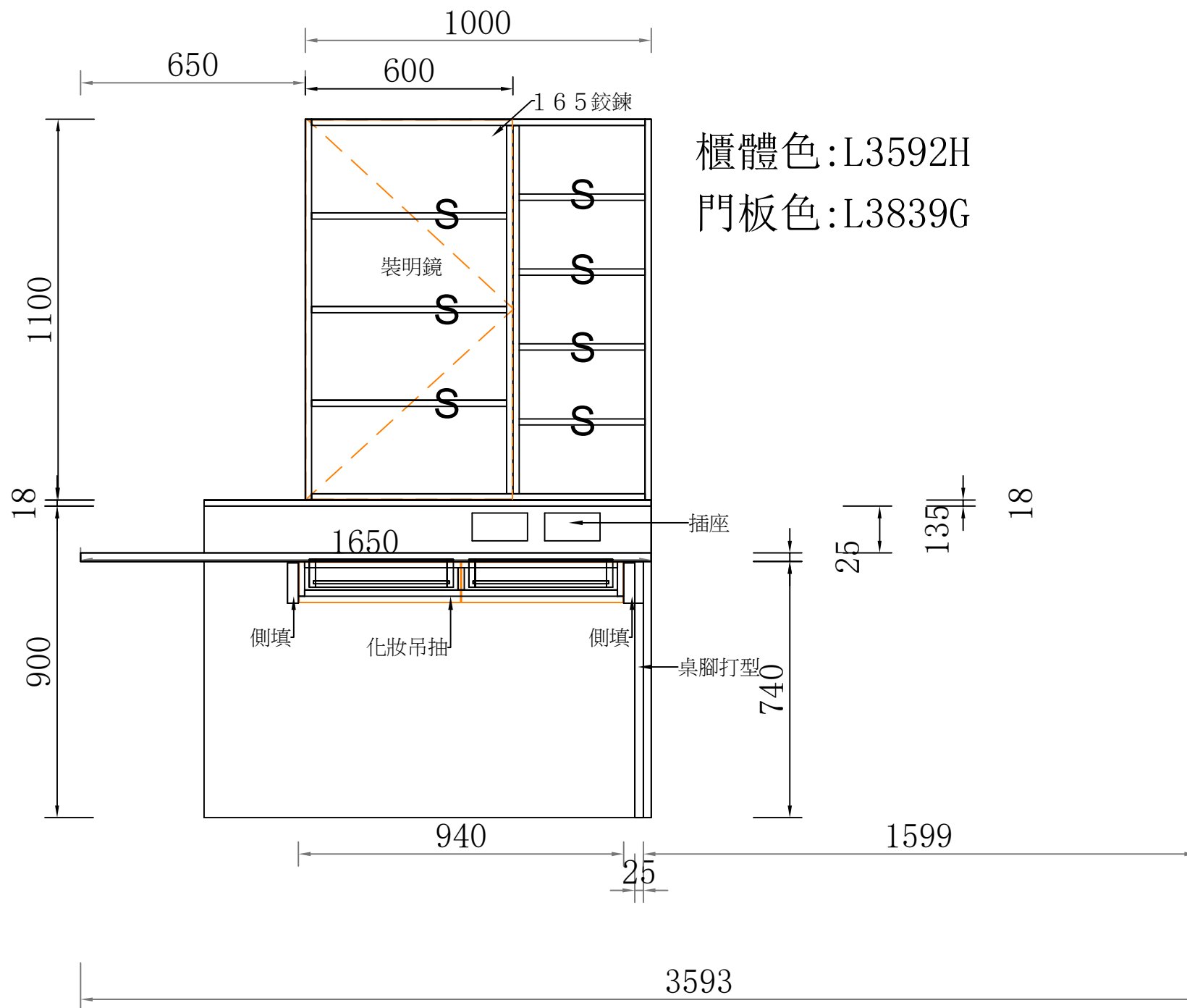
佳順大順女兒房B向立面圖
