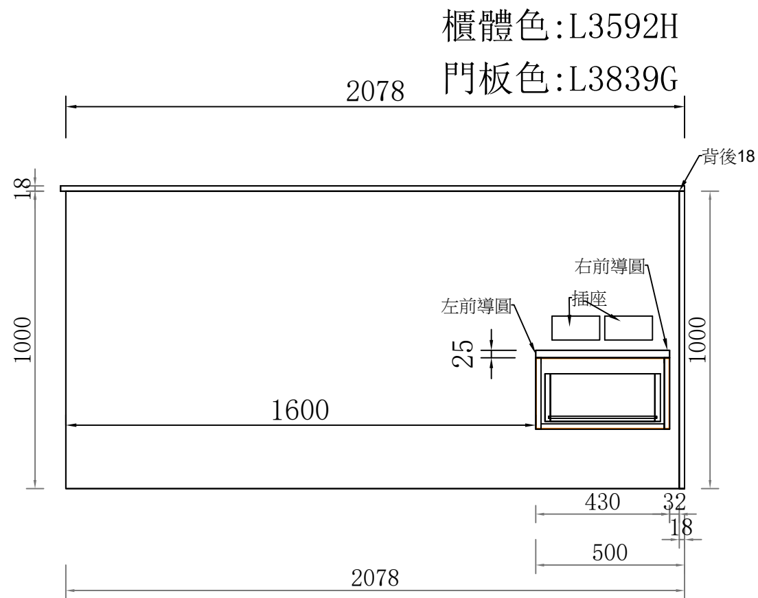
佳順大順女兒房D向立面圖
