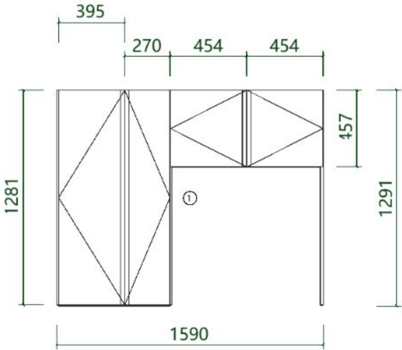
未命名A朝向门板图 (1:31.4)
