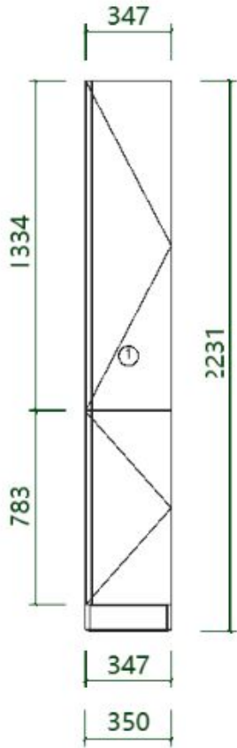
未命名A朝向门板图 (1:37.5)
