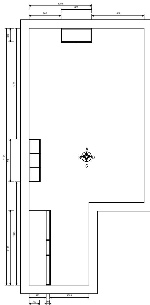
廚房頂櫃平面圖
