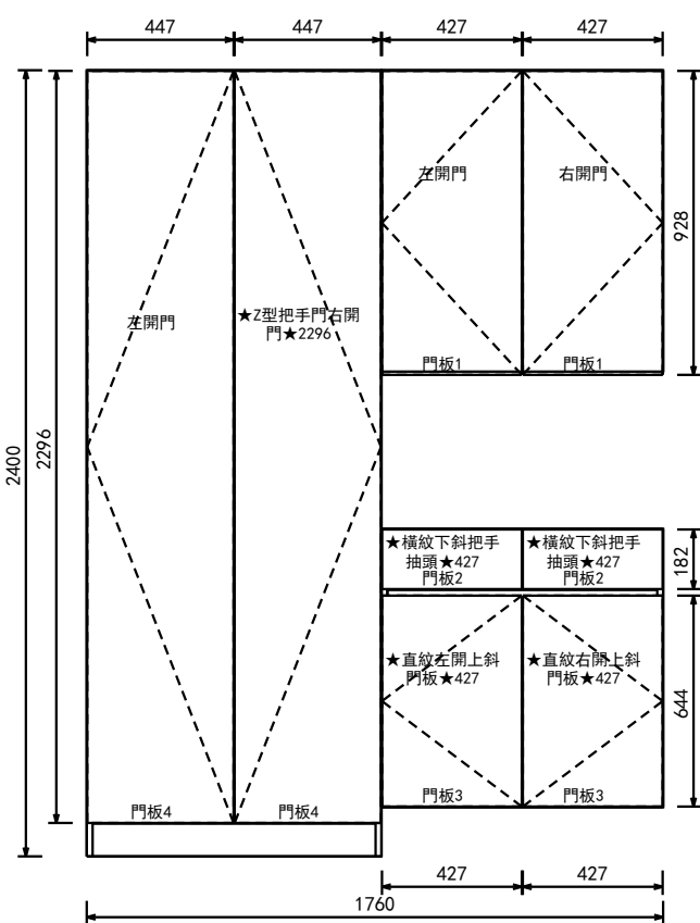
A向 立面圖
