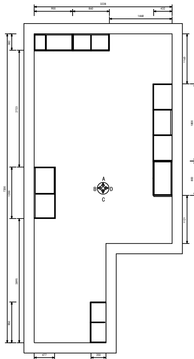
廚房地櫃平面圖
