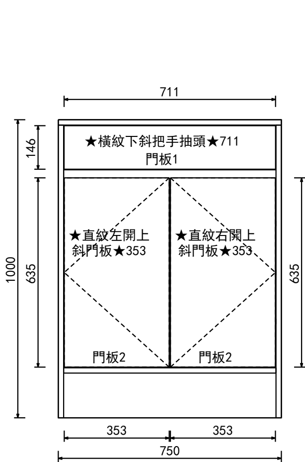
立面圖
