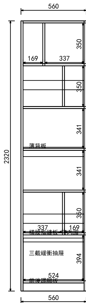
結構圖
