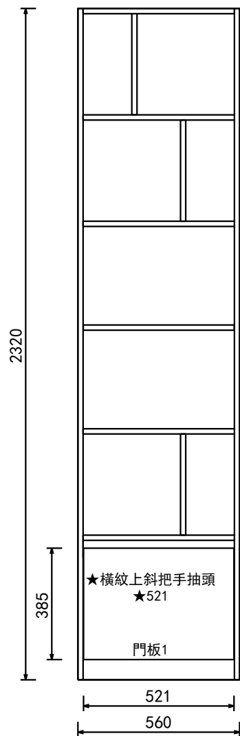
立面圖
