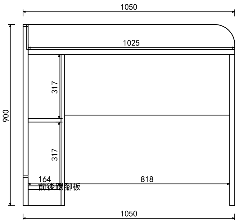
結構圖
