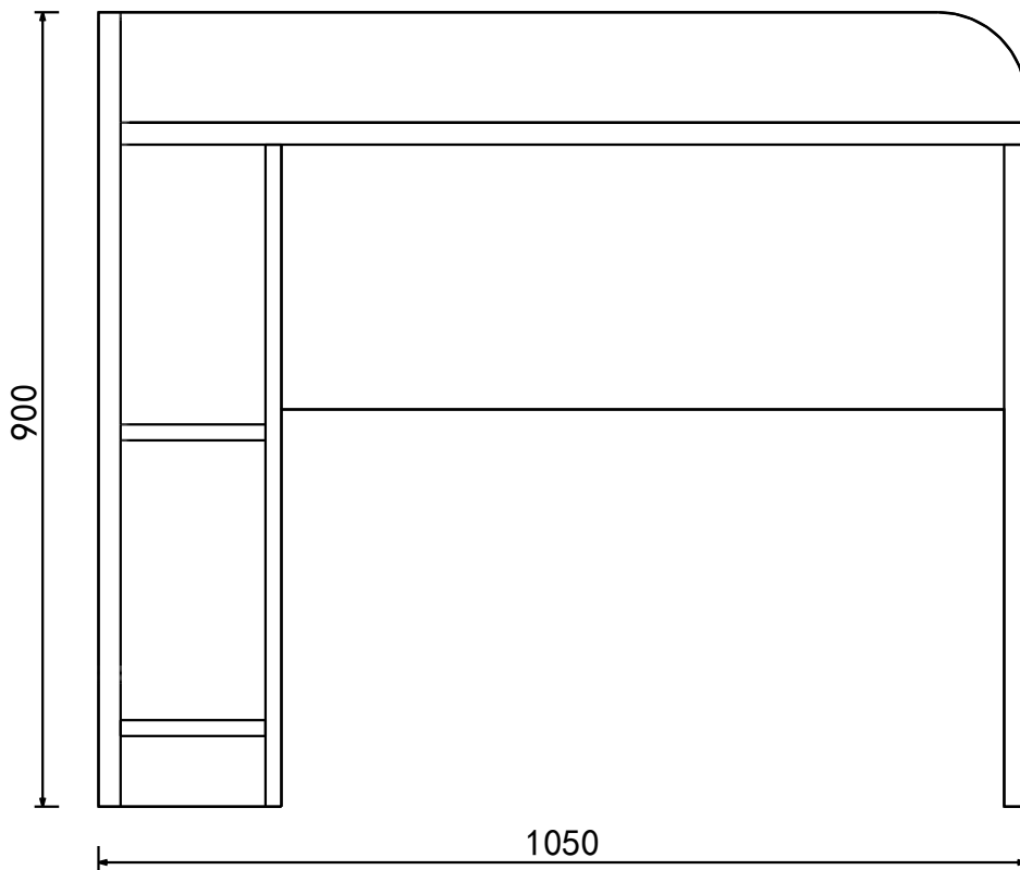
立面圖
