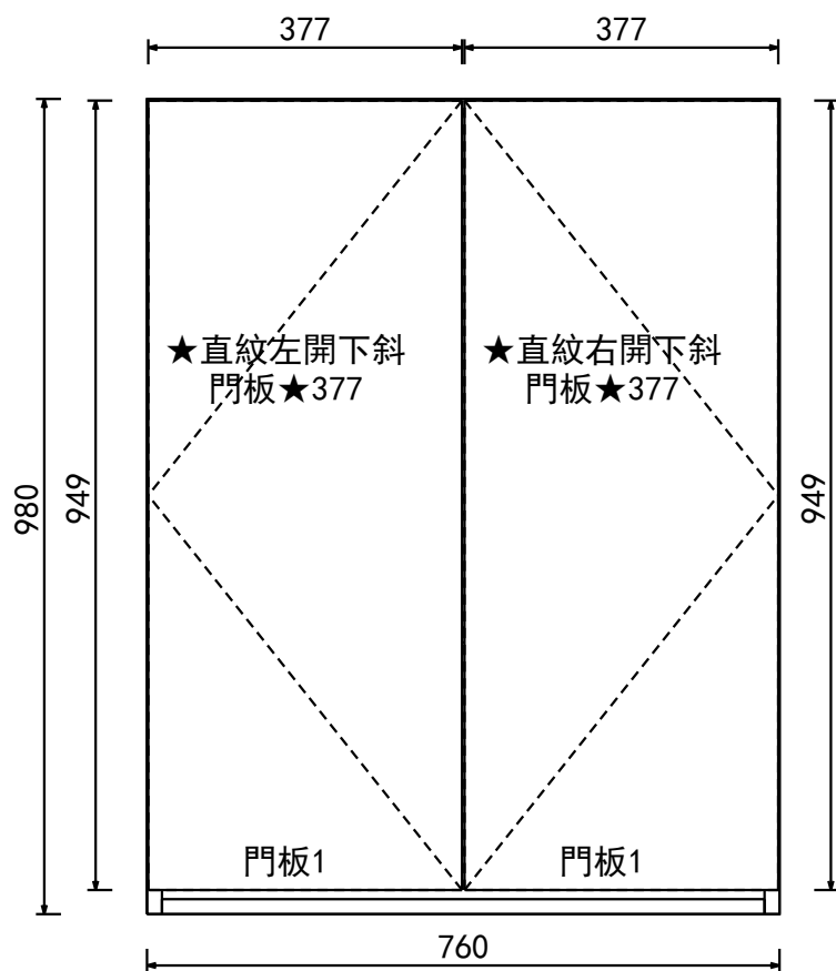
D向 立面圖
