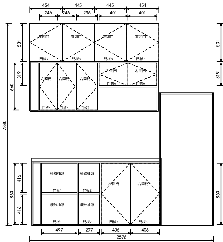
C向 立面圖
