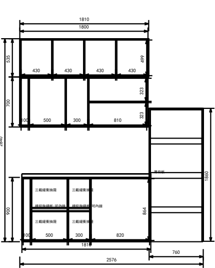
C向 結構圖
