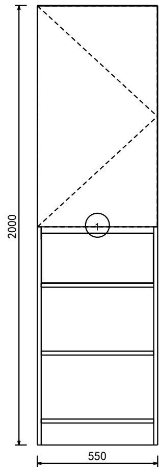
A向 外觀圖
