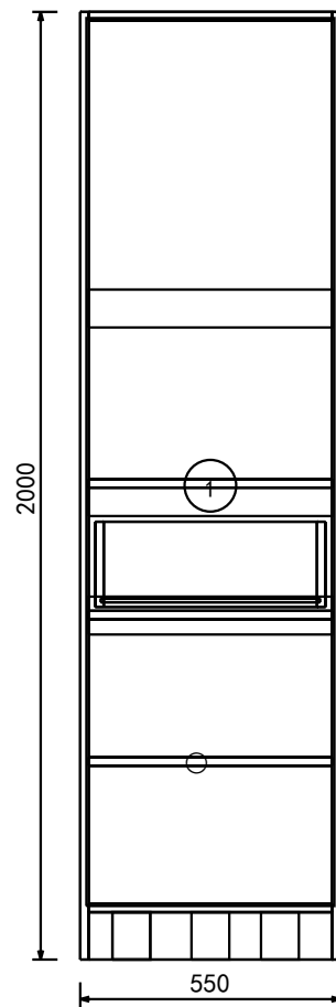
A向 結構圖
