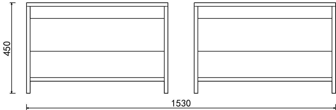
立面圖
