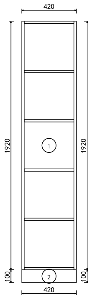
A向 外觀圖
