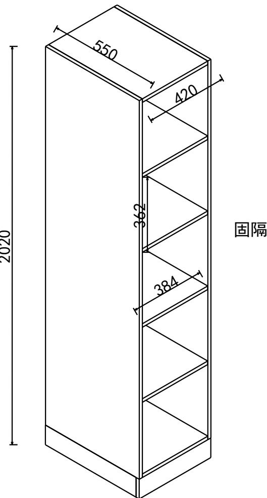
軸測圖
