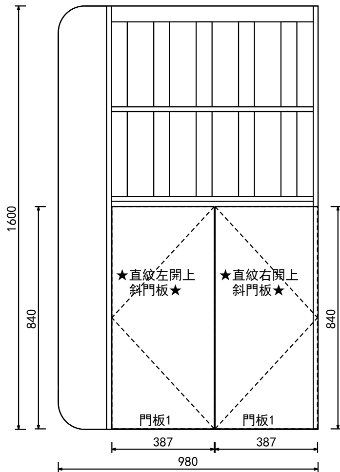
立面圖
