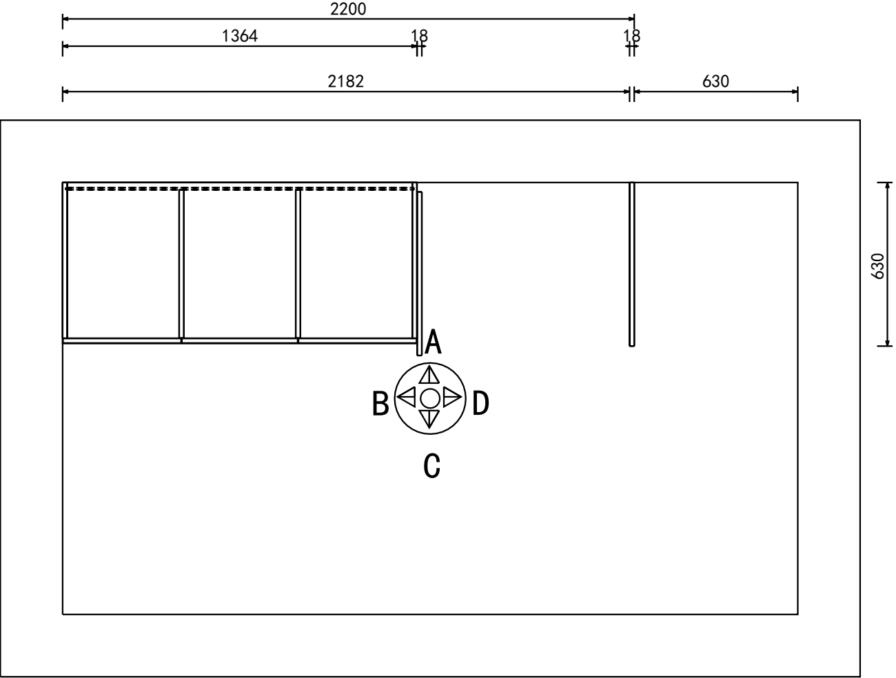
廚房地櫃平面圖
