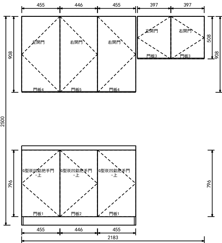
A向 立面圖
