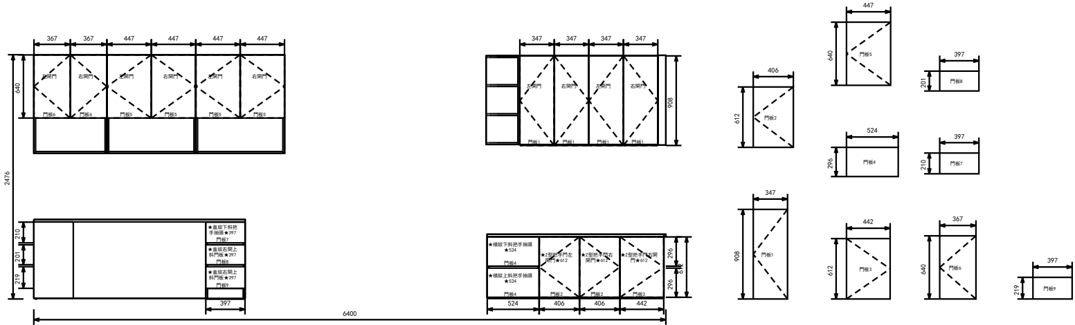
A向 立面圖
