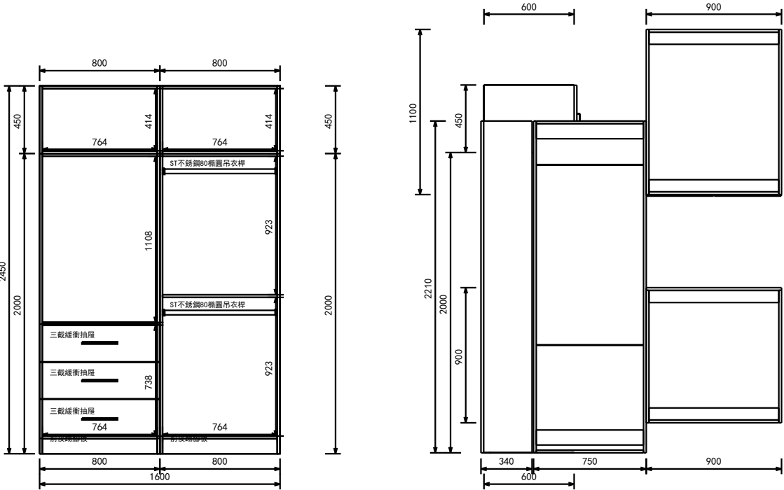
C向 結構圖
