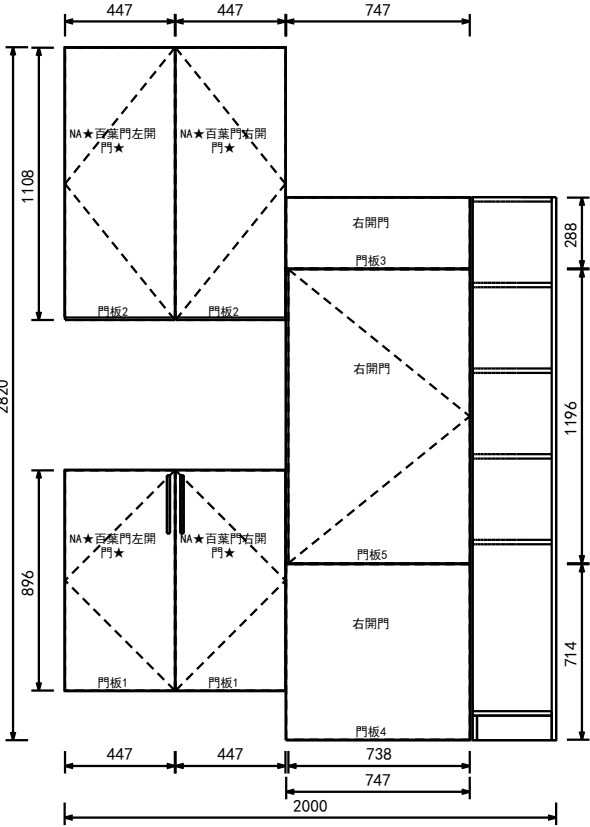
D向 立面圖
