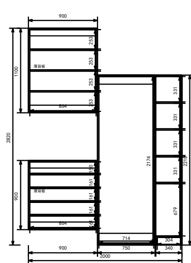
D向 結構圖
