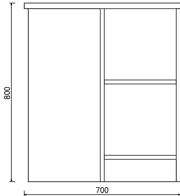
B向 立面圖
