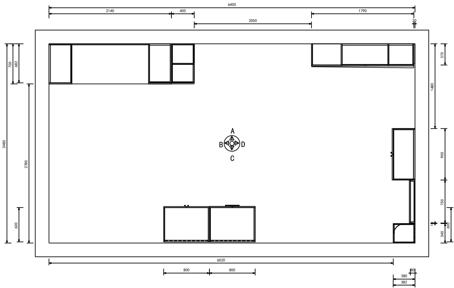
主臥地櫃平面圖
