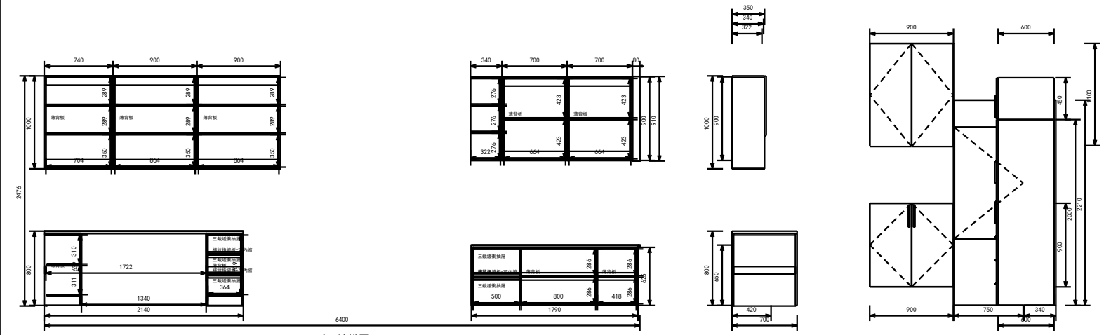
A向 結構圖
