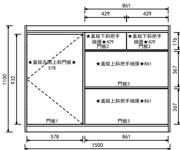
立面圖
