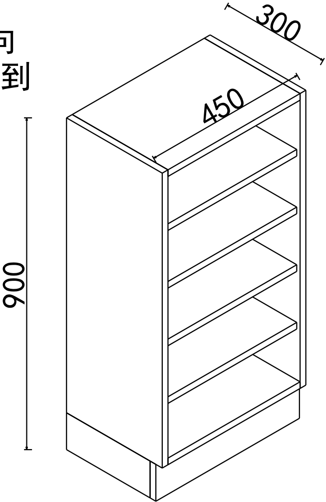
軸測圖
