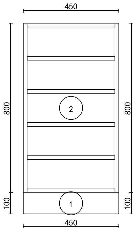
A向 外觀圖
