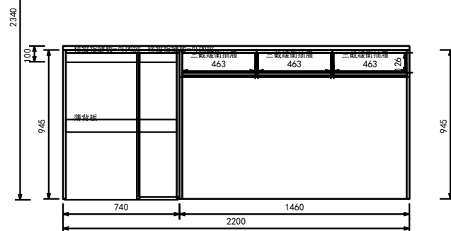
B向 結構圖
