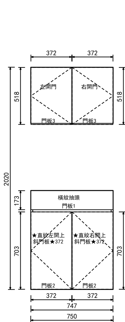
D向 立面圖
