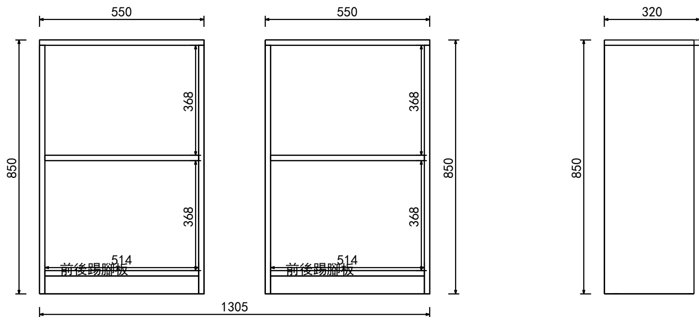
結構圖
