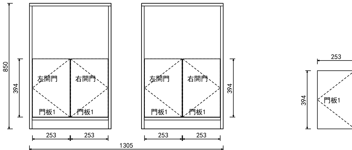
立面圖
