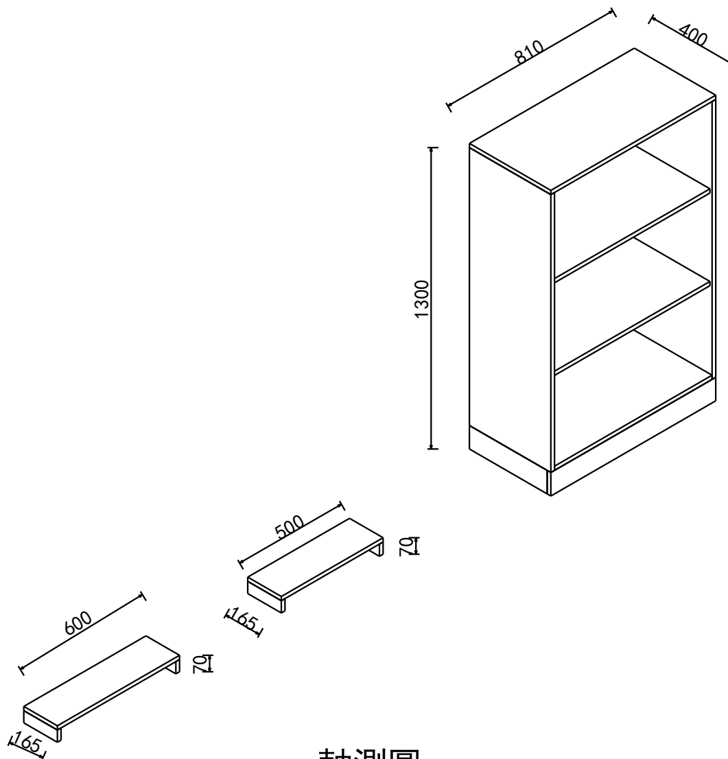
軸測圖
