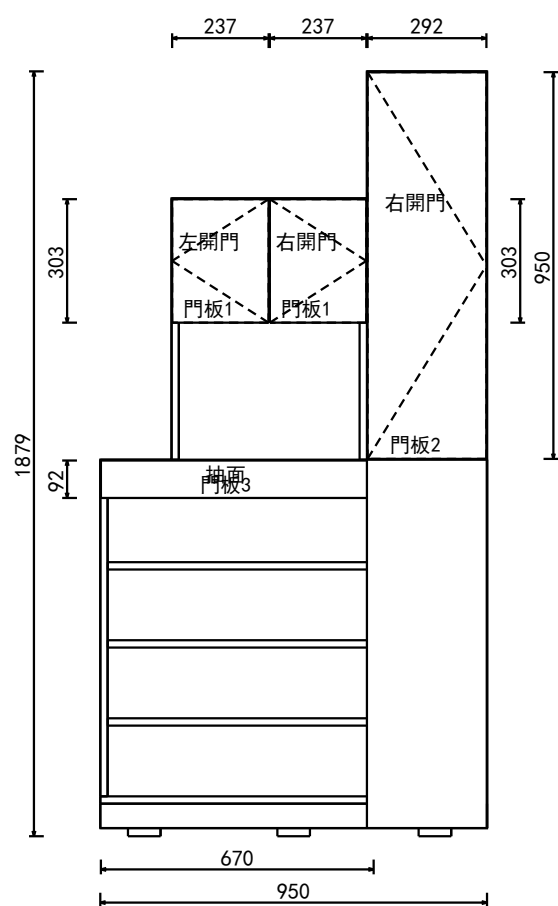
立面圖
