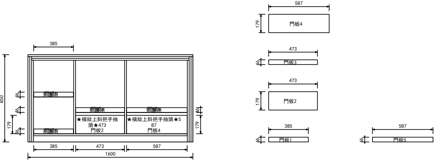
立面圖
