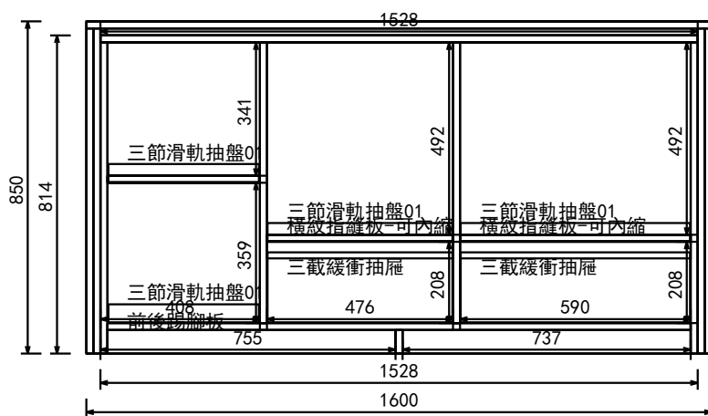
結構圖
