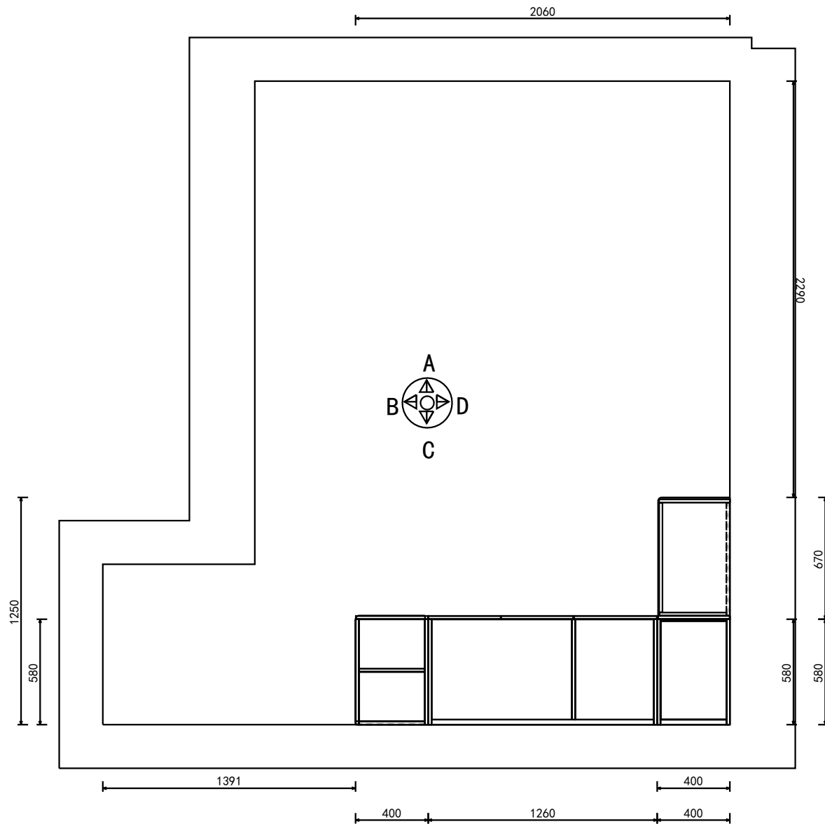
主臥地櫃平面圖
