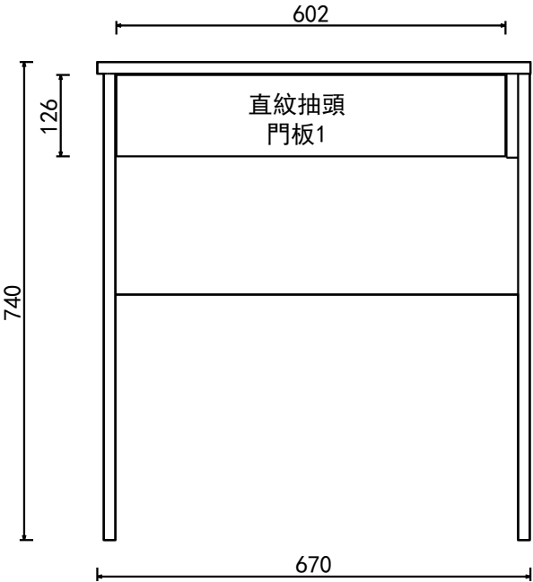
D向 立面圖
