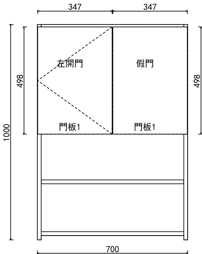
A向 立面圖
