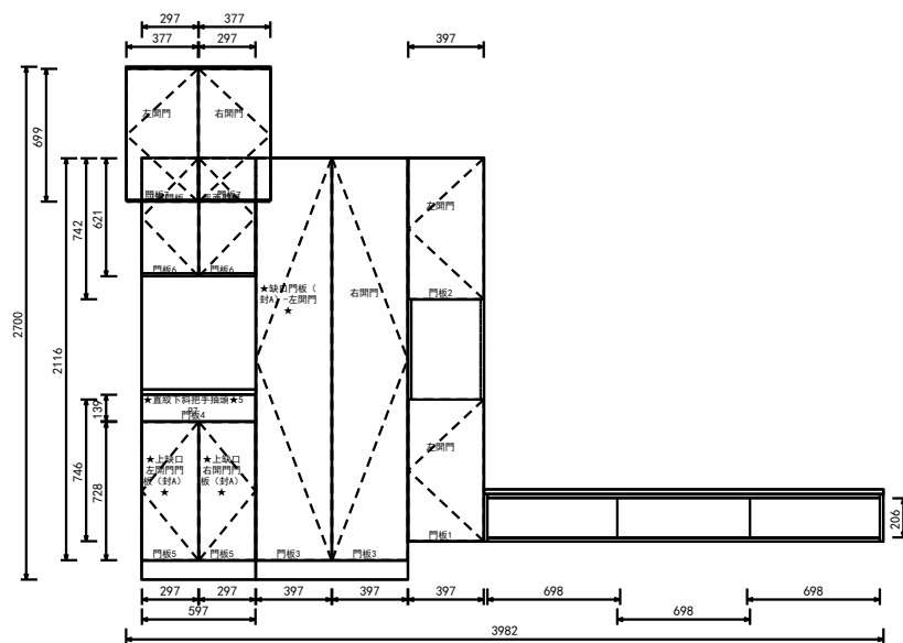
B向 立面圖
