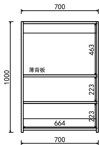
A向 結構圖
