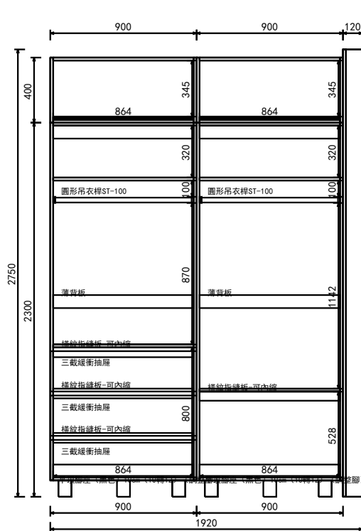
C向 結構圖
