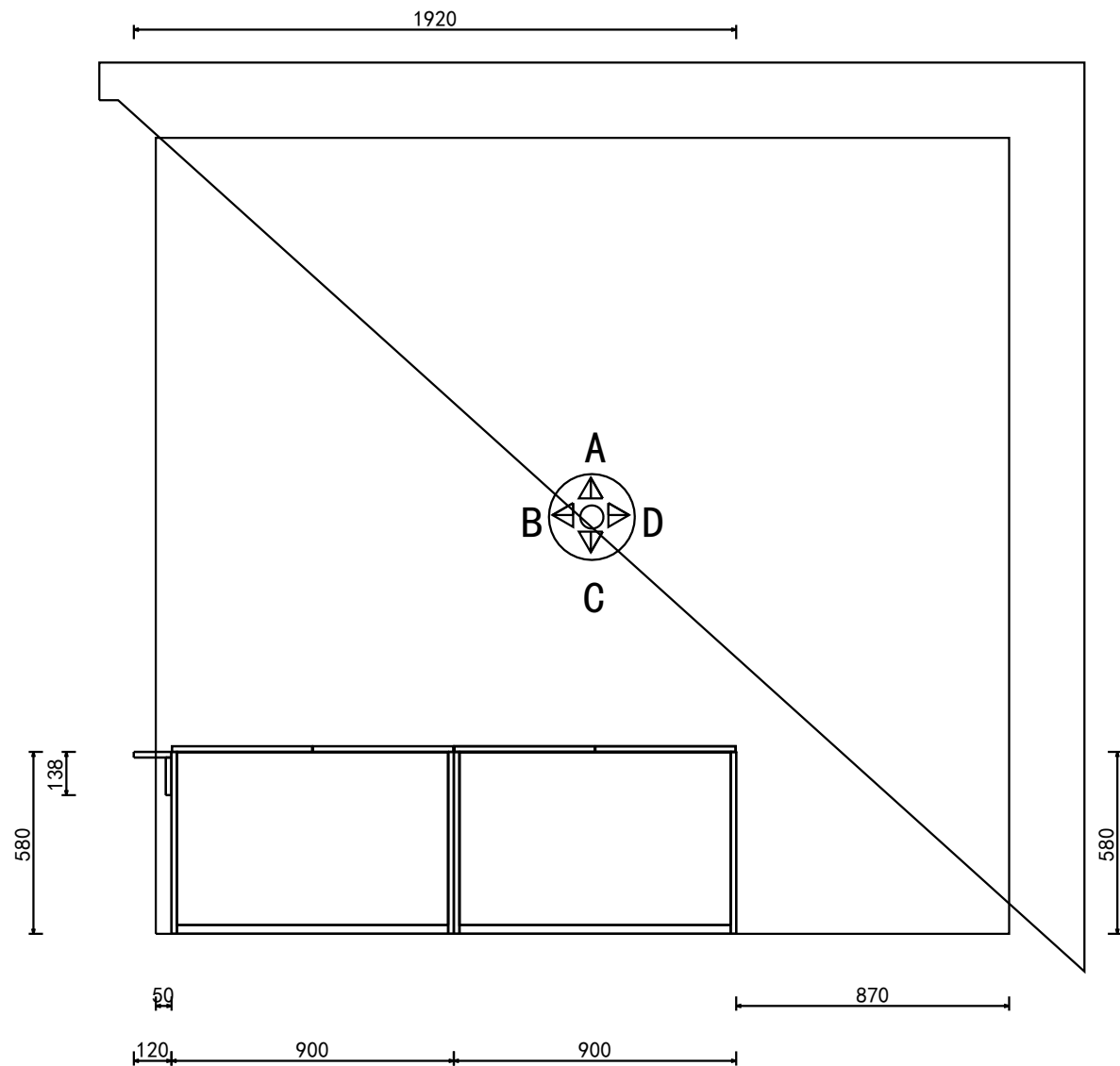
臥室地櫃平面圖
