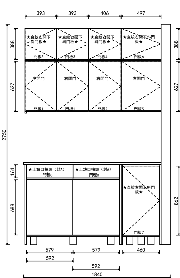
D向 立面圖
