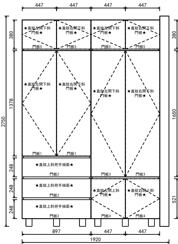
C向 立面圖
