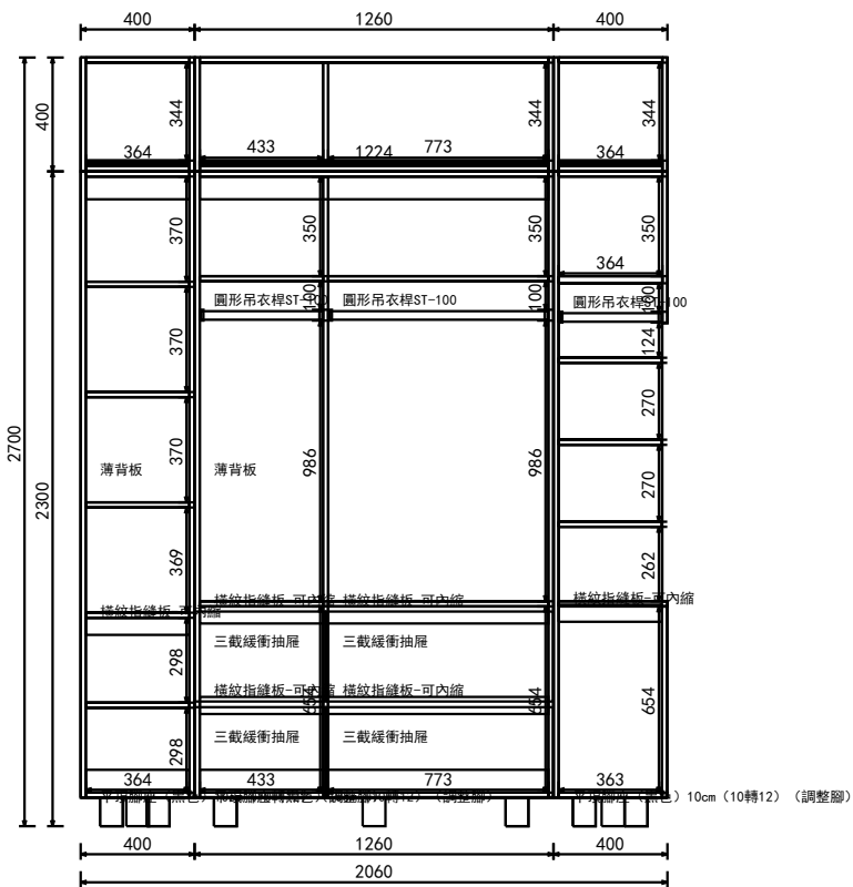
C向 結構圖
