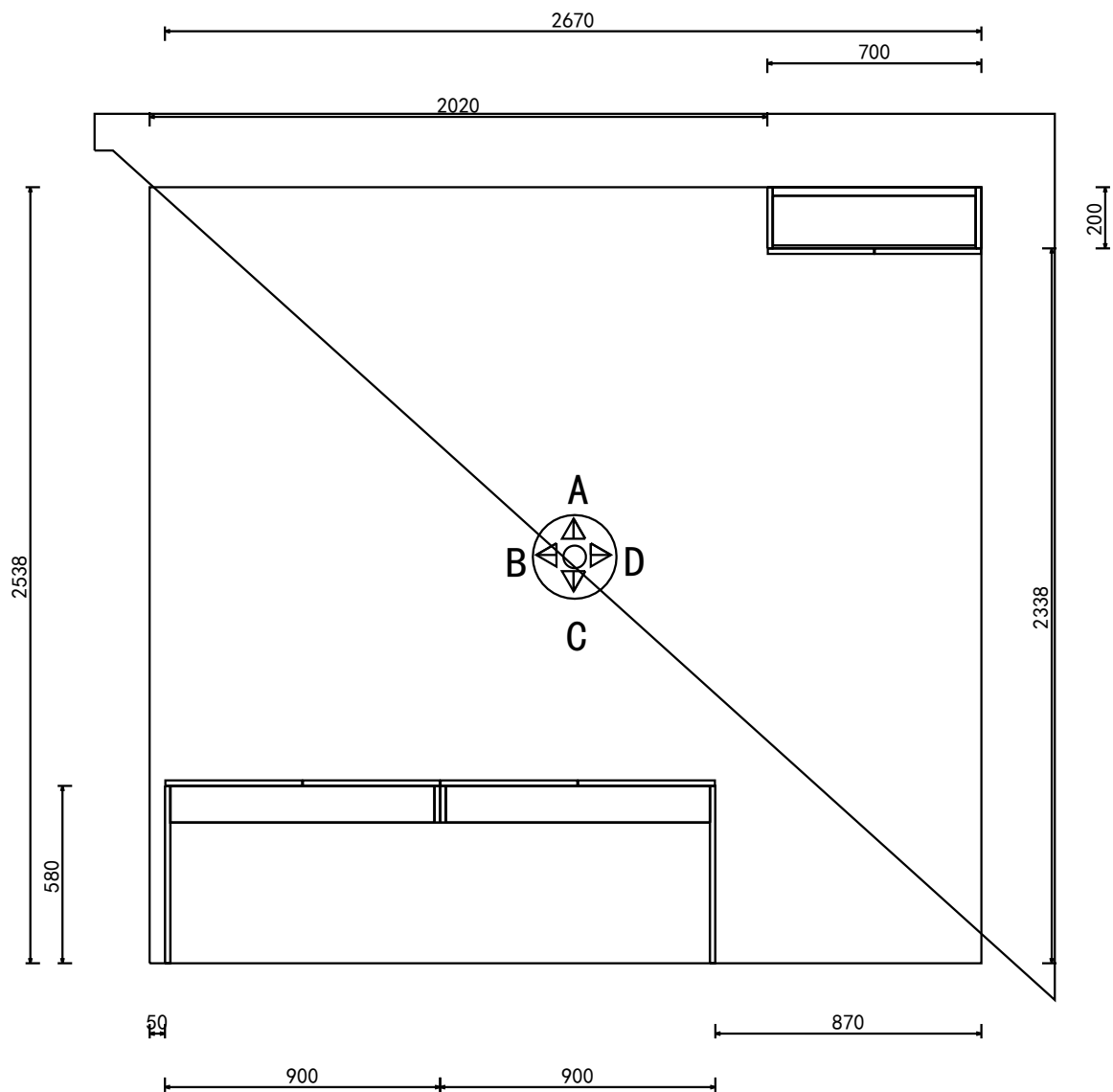
臥室頂櫃平面圖
