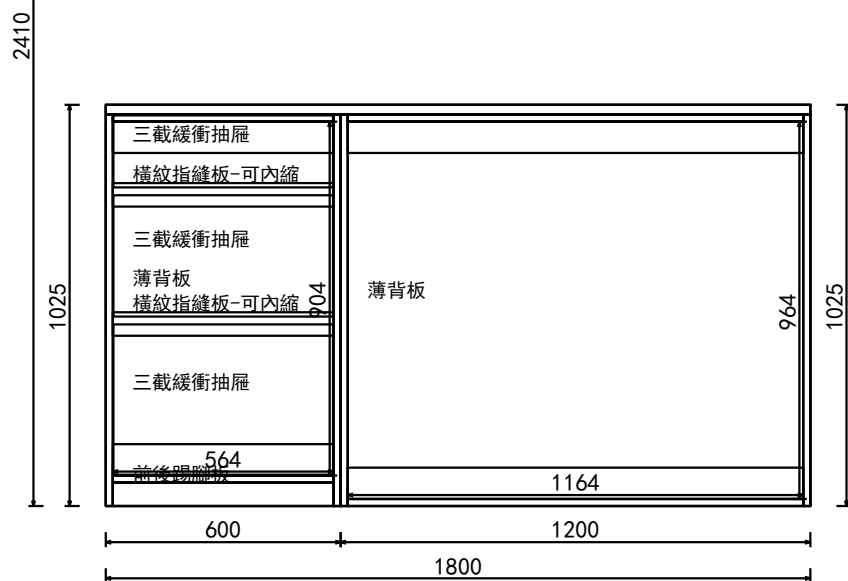
結構圖
