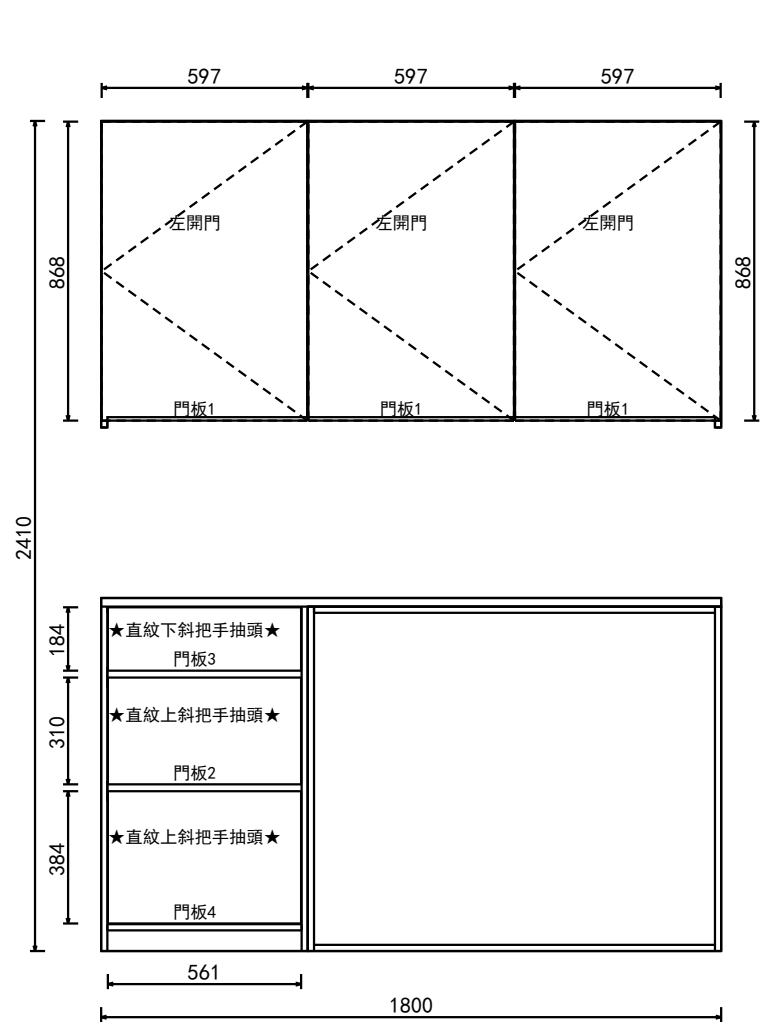
立面圖
