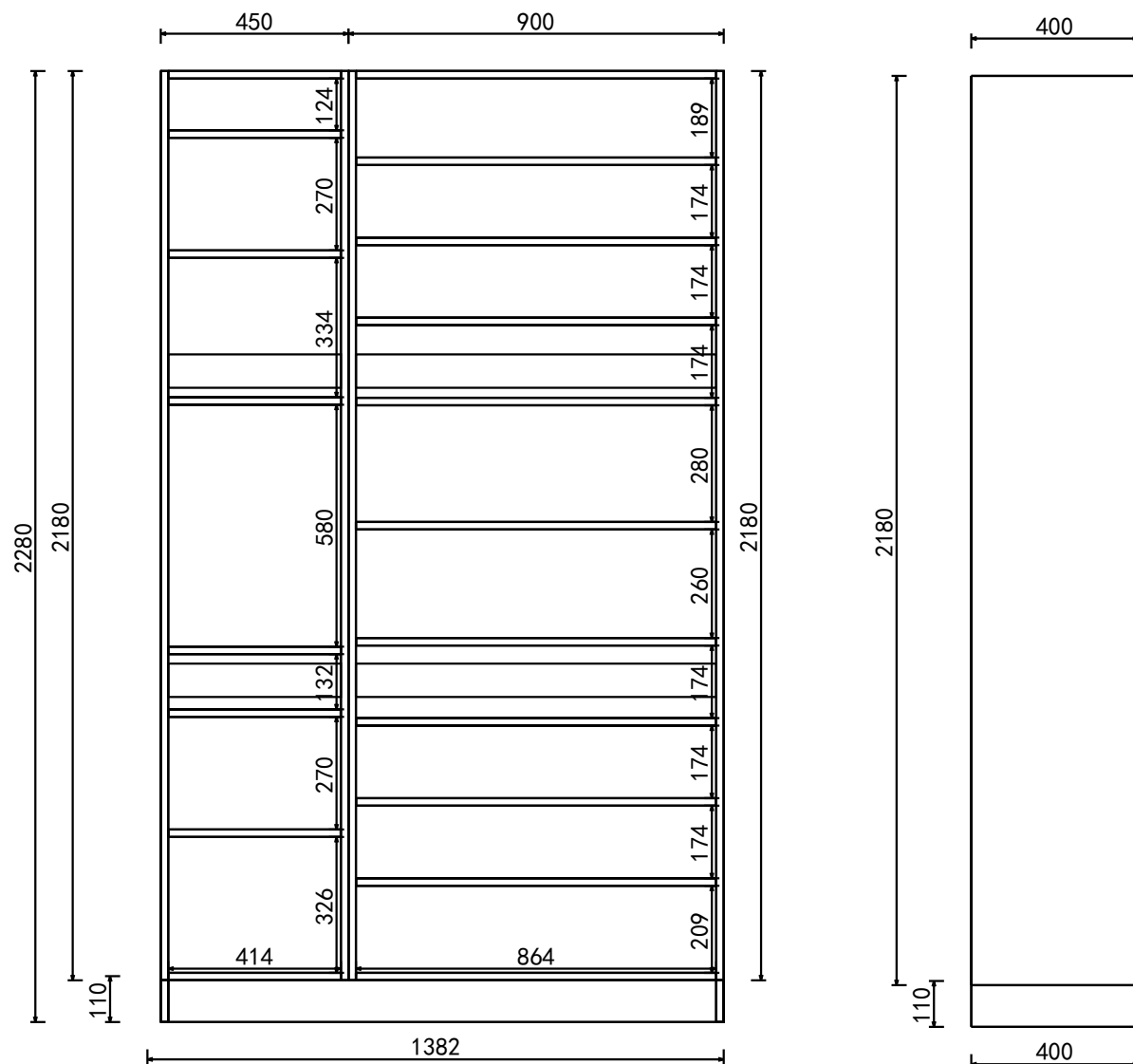
結構圖
