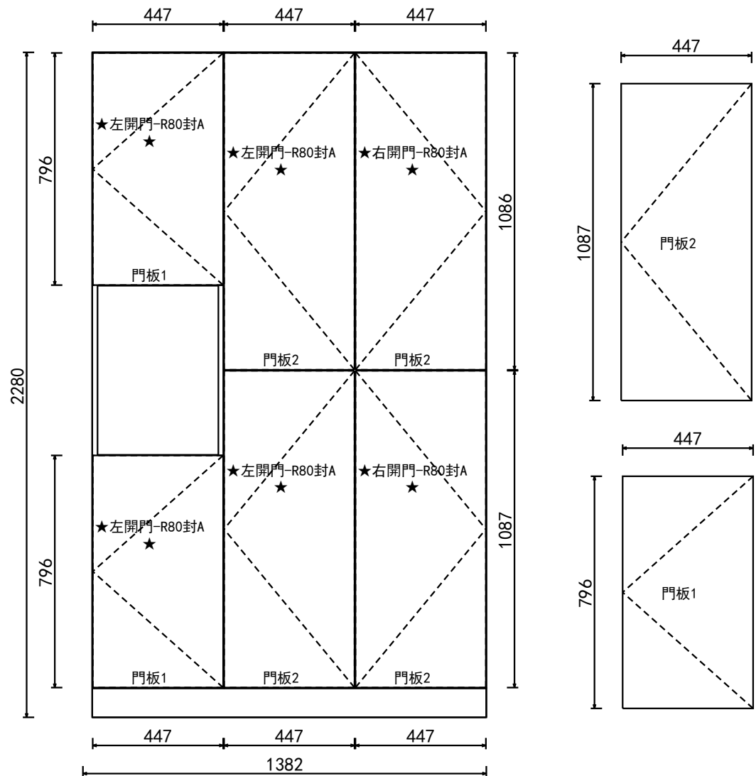
立面圖
