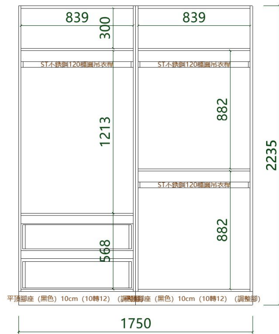
主臥 A朝向結構圖 (1:19.7)
