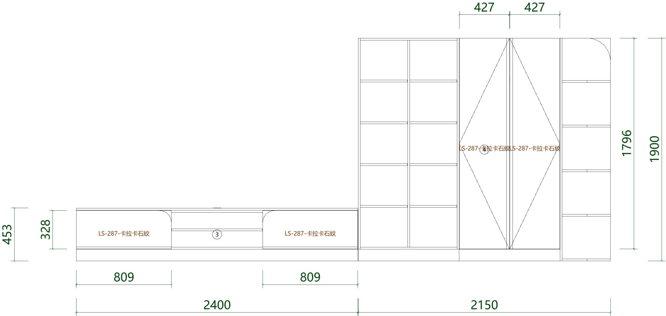
客廳家廚房 B朝向門板圖 (1:13)
