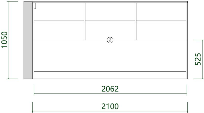
次臥1 A朝向門板圖 (1:18)
