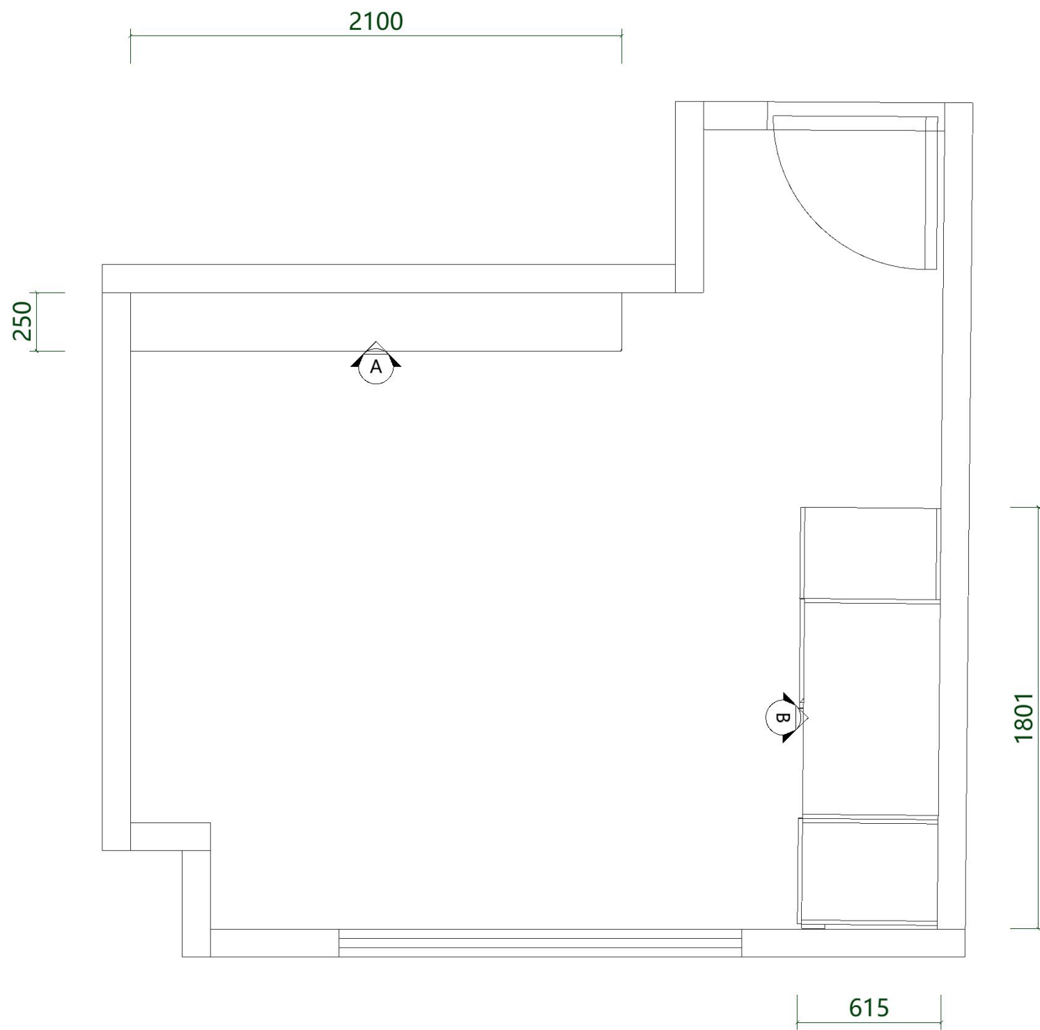
次臥1 地櫃平面圖 (1:15.8)
