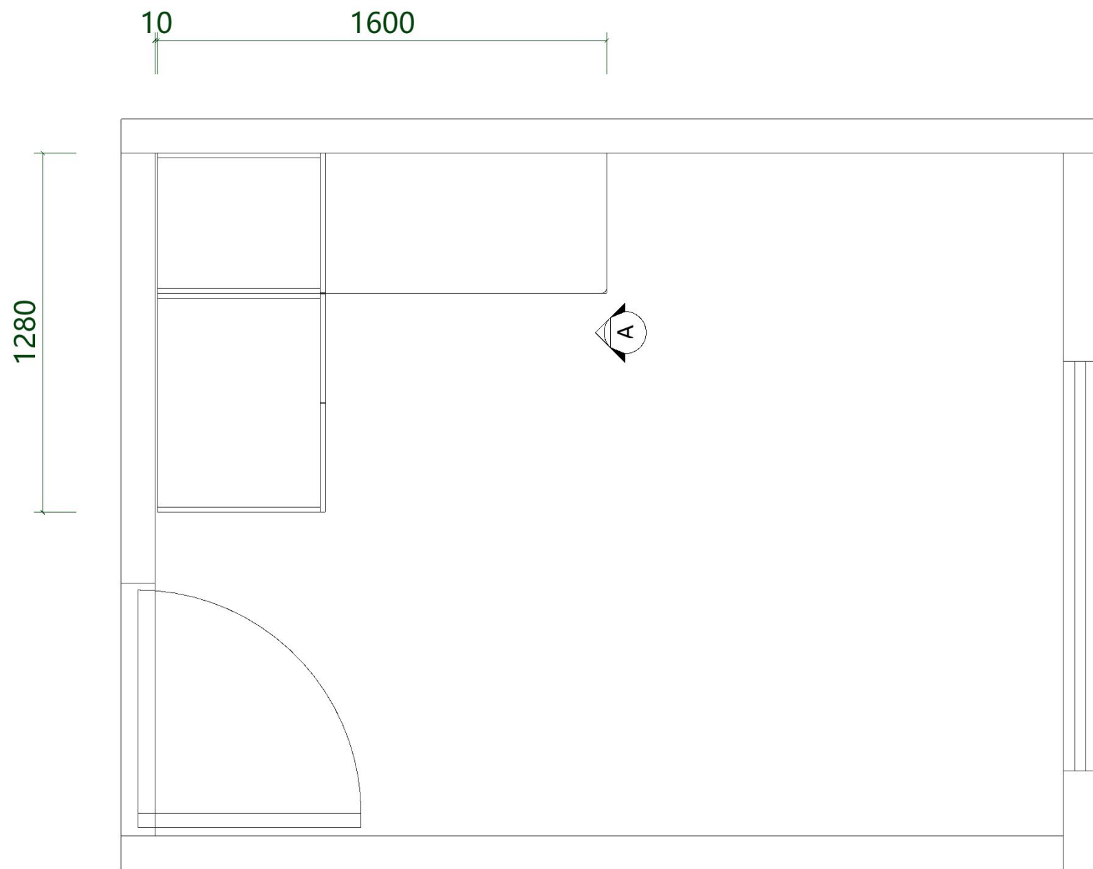
次臥2 地櫃平面圖 (1:13)
