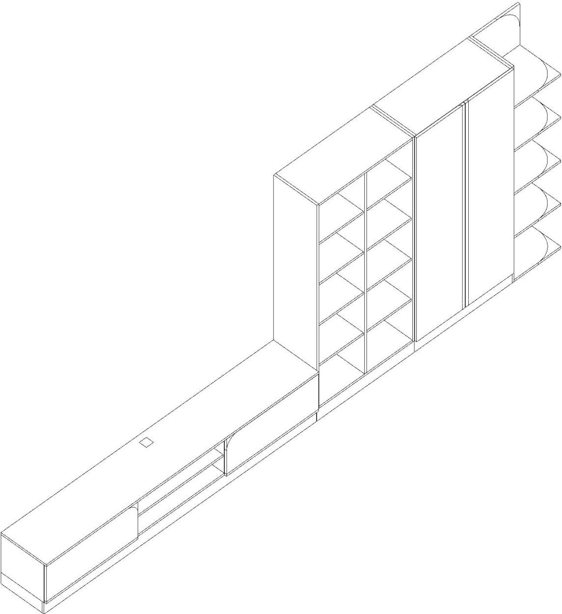
客廳家廚房 軸測圖 (1:16.2)
