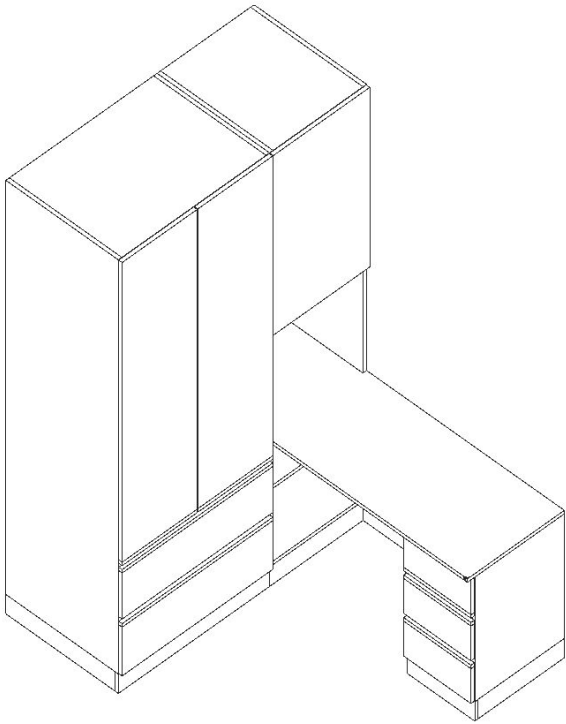
次臥2 A朝向軸測圖 (1:19.3)
