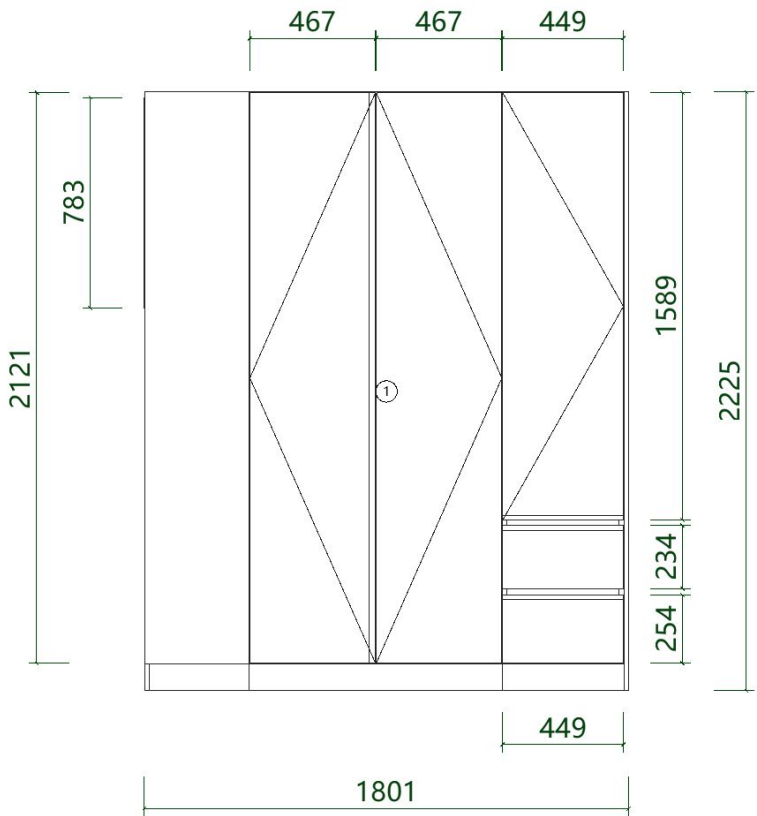
次臥1 B朝向門板圖 (1:19.7)
