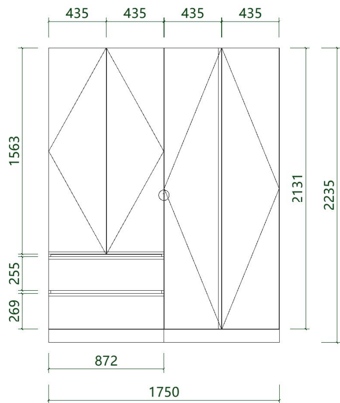
主臥 A朝向門板圖 (1:19.7)
