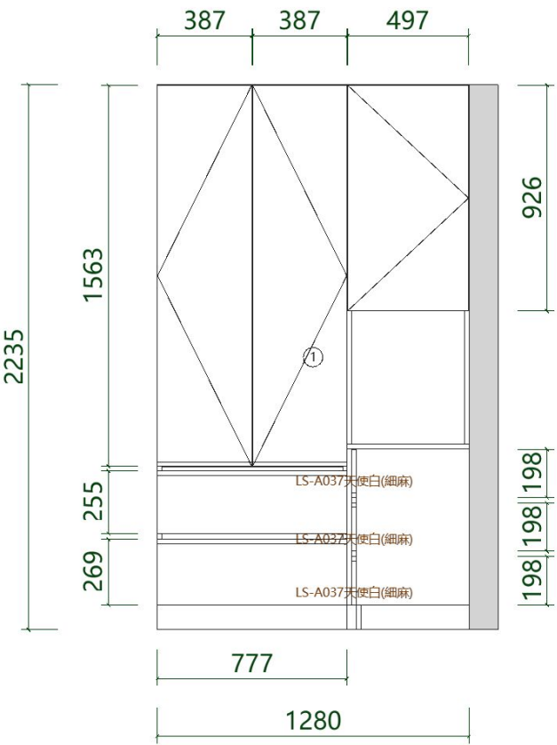
次臥2 A朝向門板圖 (1:19.3)
