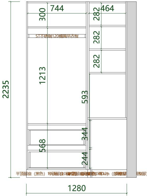
次臥2 A朝向結構圖 (1:19.3)
