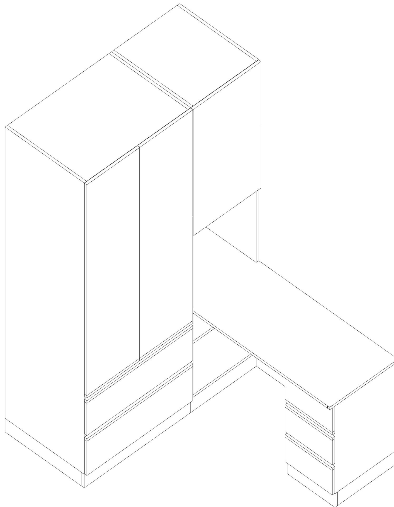
次臥2 軸測圖 (1:8.2)
